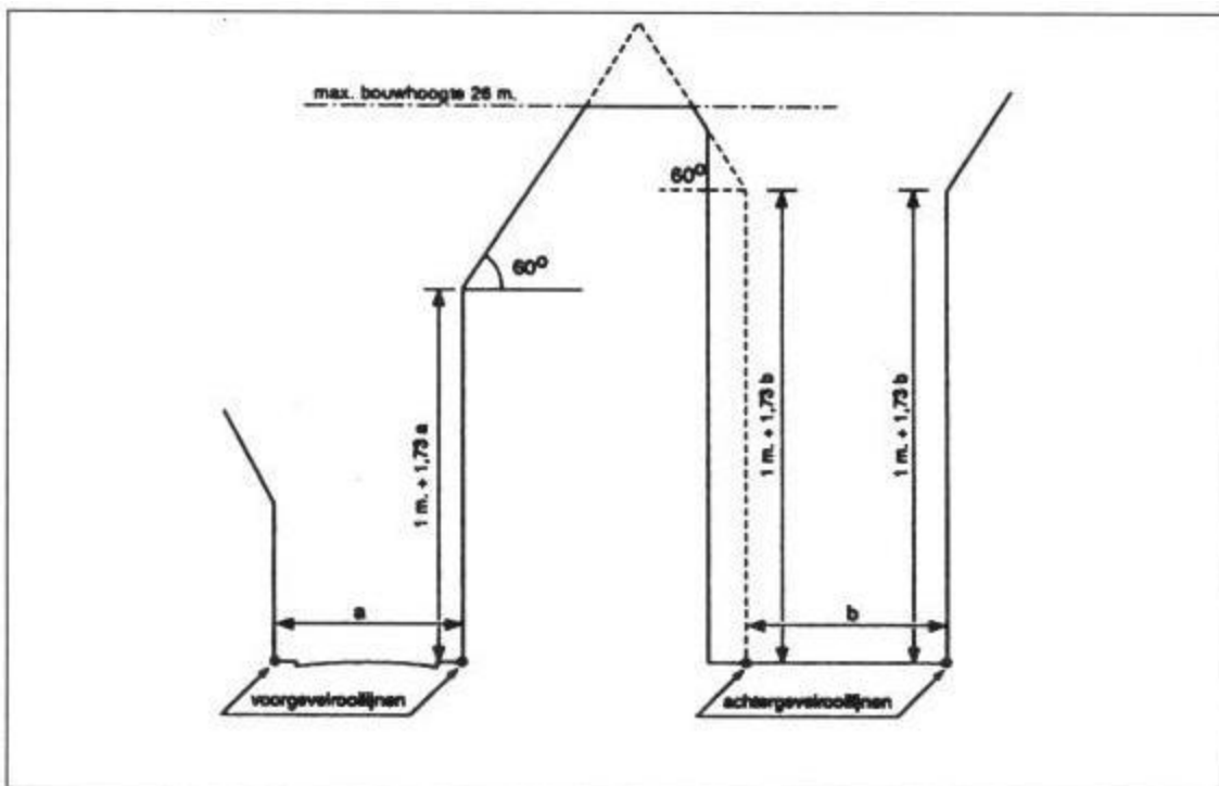
Figuur 14 Bouwhoogte in voor- en achtergevelrooilijn en daartussen. Maximum bouwhoogte (artikelen 2.5.20, 2.5.21, 2.5.23 en 2.5.24)
