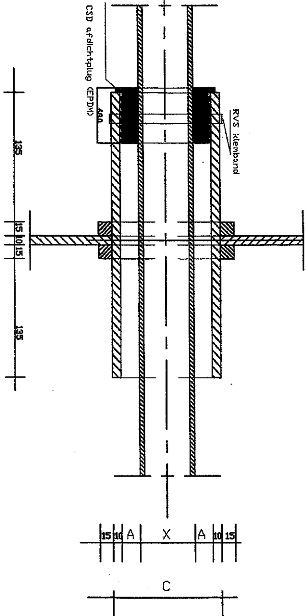
ZIJAANZICHT / LANGSDDOORSNEDE
