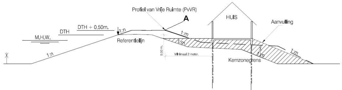
Figuur 7: binnendijs bouwen bij regionale waterkeringen
