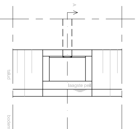
Bovenaanzicht
