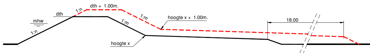
Figuur 2: Piping is maatgevend
