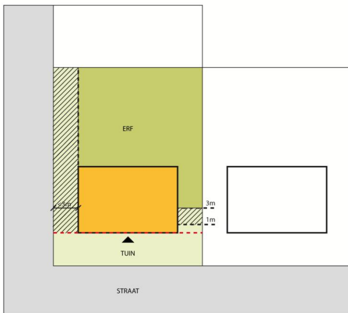
Bouwvlak <math>< 3m</math> tot openbaar gebied
