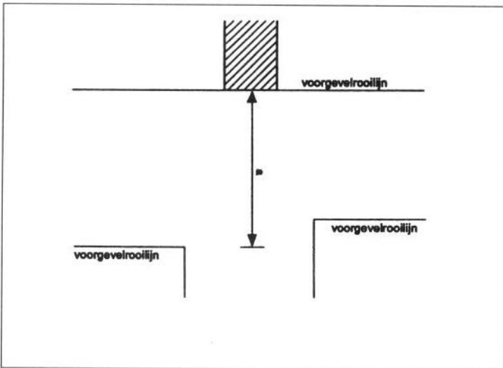
Figuur 16 Bouwhoogte in de voorgevelrooilijn (artikelen 2.3.17, derde lid, tweede alinea)
