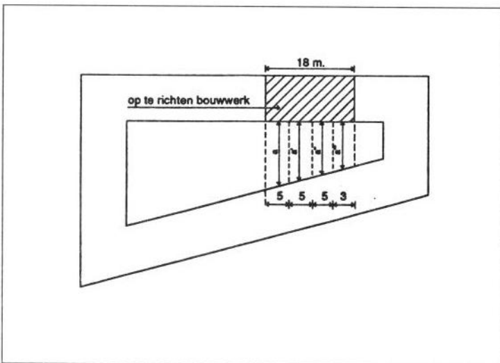
Figuur 17 Bouwhoogte in de achtergevelrooilijn (artikelen 2.3.18, tweede lid, eerste alinea)
