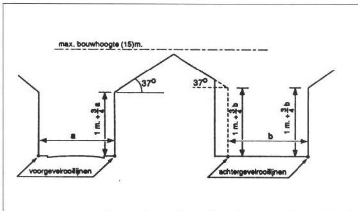
Figuur 13 Bouwhoogte in voor- en achtergevelrooilijn en daartussen. Maximum bouwhoogte (artikelen 2.3.17, 2.3.18, 2.3.19 en 2.3.20). Buiten de bebouwde kom
