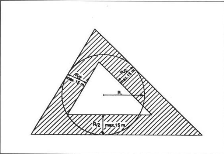
Figuur 5 Ligging van de achtergevelrooilijn (artikel 2.3.8, eerste lid, onder a)
