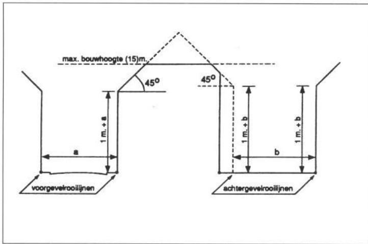
Figuur 12 Bouwhoogte in voor- en achtergevelrooilijn en daartussen. Maximum bouwhoogte (artikelen 2.3.17, 2.3.18, 2.3.19 en 2.3.20). Binnen de bebouwde kom
