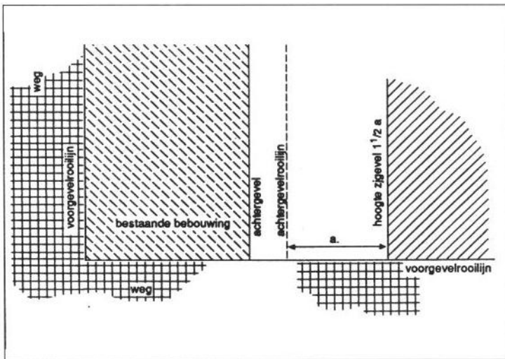
Figuur 19 Hoogte van een zijgevel tegenover een achtergevelrooilijn (artikelen 2.3.19)
