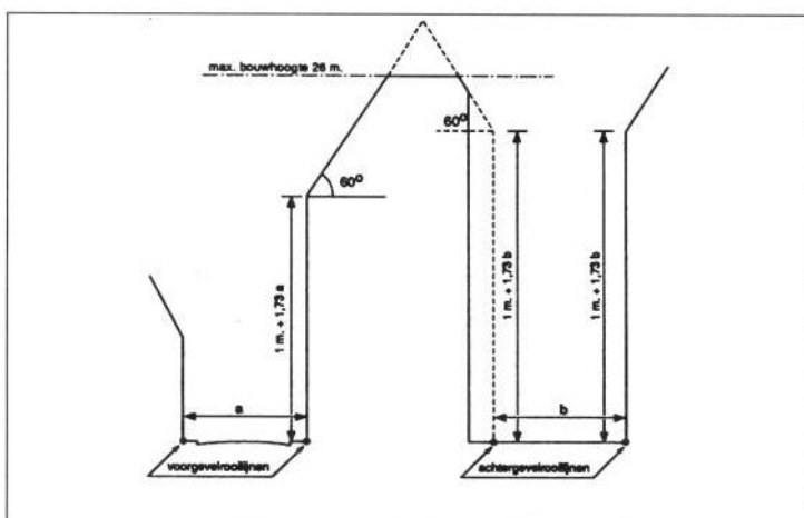
Figuur 14 Bouwhoogte in voor- en achtergevelrooilijn en daartussen. Maximum bouwhoogte (artikelen 2.3.17, 2.3.18, 2.3.19 en 2.3.20, alternatief 2). Binnen grootstedelijke delen van de bebouwde kom
