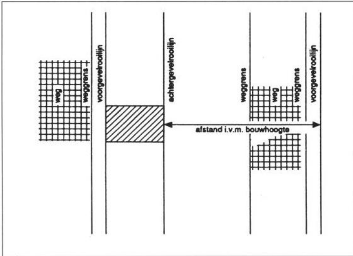
Figuur 18 Bouwhoogte in de achtergevelrooilijn (artikelen 2.3.17, tweede lid, tweede alinea)
