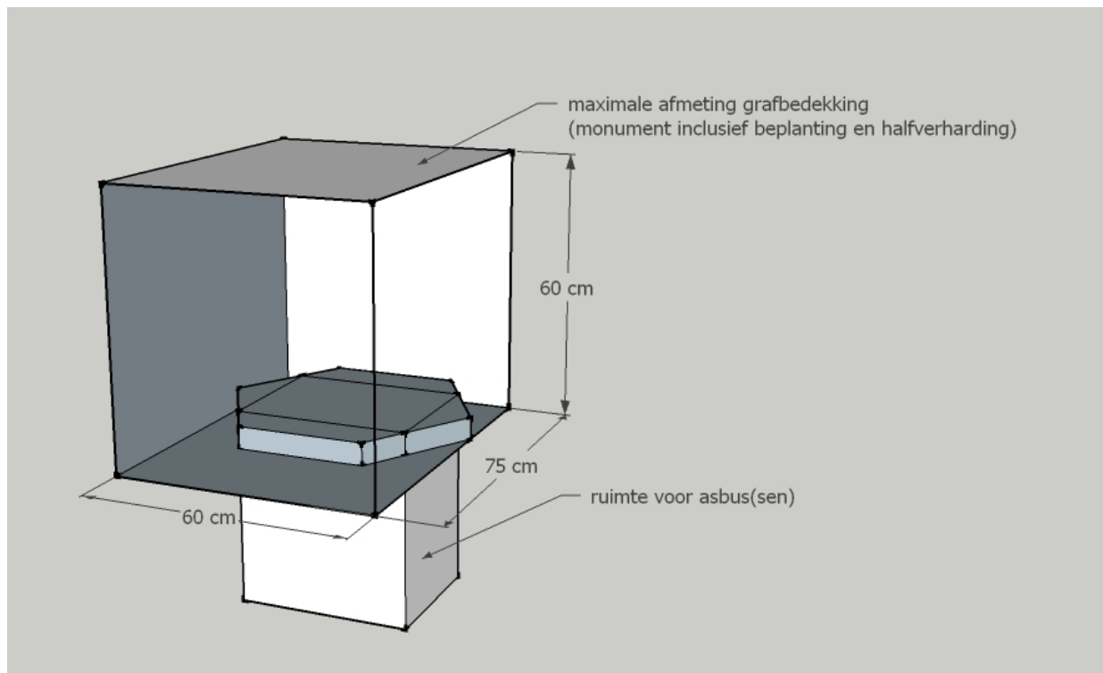
Afbeelding 3: afmetingen bij een urnengraf
