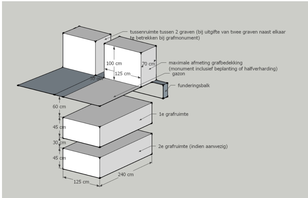
Afbeelding 1: afmetingen bij een particulier en algemeen graf
