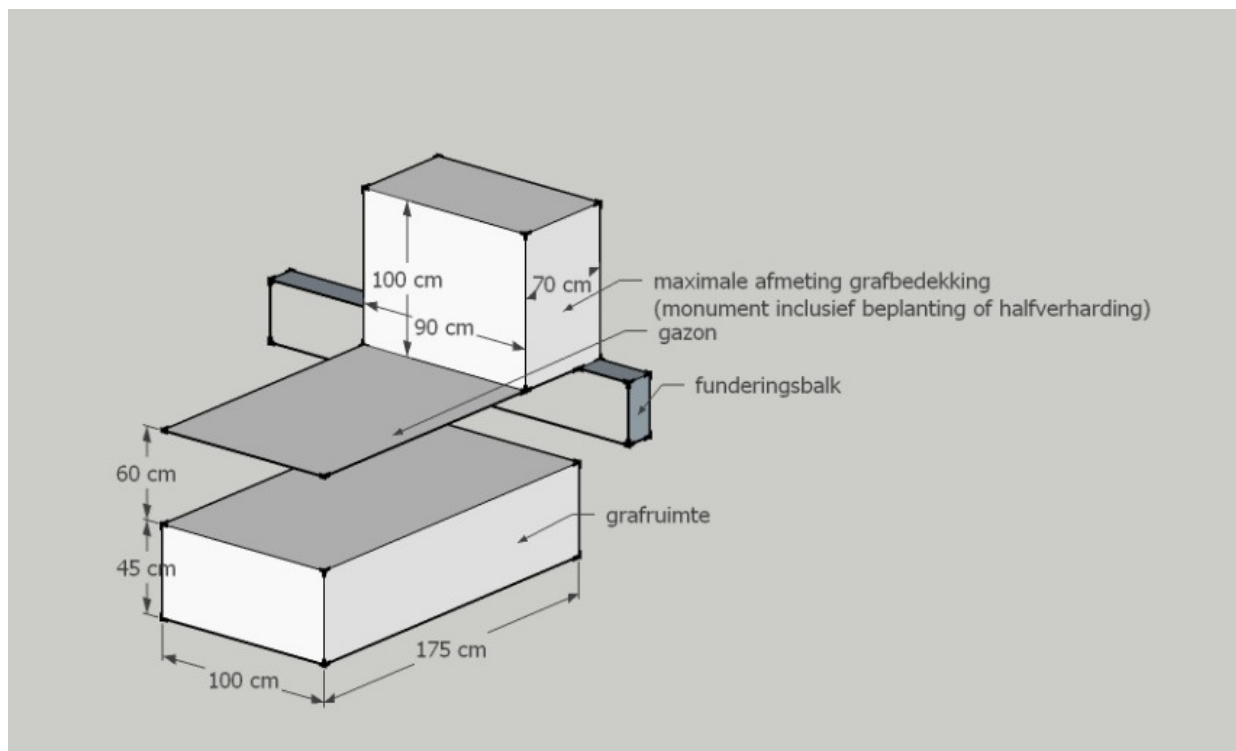
Afbeelding 2: afmetingen bij een kindergraf
