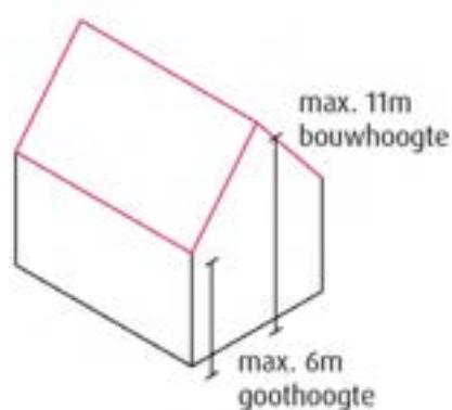
Afbeelding 234. Basis bouwhoogte.
