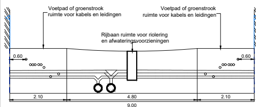
Woonstraat met bebouwing op erfgrans aan beide zijden
