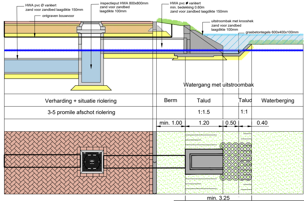
Profiel 14: Uitstrooprofiel
