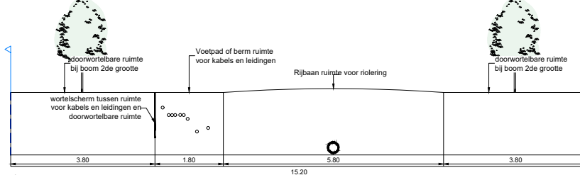
Lint met bomen 2de grootte aan een zijde van de weg met watergang
