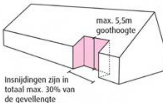
Afbeelding 101. Principes insnijdingen.
