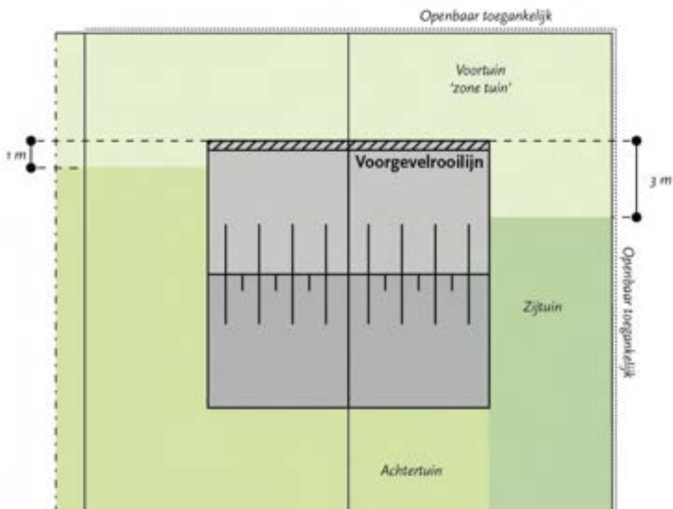
Afbeelding 43. Principetekening met specificatie tuin en minimale afstand achter de Voorgevelrooilijn
