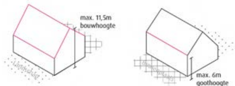
Afbeelding 149. Bouwhoogtes Poortgebouw.
