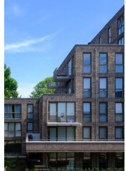
Subtiële variatie in gevelritmiek versterkt de leesbaarheid van de verschillende volumes. Strokentoren, Haarlem (Hoogveen Architecten)
