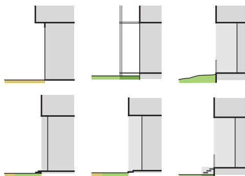
Indicatieve principedoorssneden van mogelijke aanhechtingen van landschap op vloerniveau.
