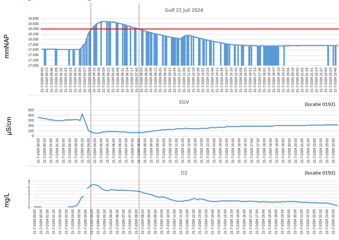
Figuur 2.4 Waterstand en waterkwaliteit in de Gender bij bui 21 juli 2024. De EGV (elektrische geleidbaarheid) daalt sterk tot een waarde tussen de 50-100 \mu\text{S}/\text{cm} , hetgeen in de range ligt van afstromende neerslag. De zuurstofconcentratie stijgt eerst fors tot 7 mg/l door de aanvoer van zuurstofrijk water uit verbeterd gescheiden stelsels en riooloverstorten, om daarna langzaam te dalen doordat het in het overgestorte water aanwezige BZV wordt omgezet.
