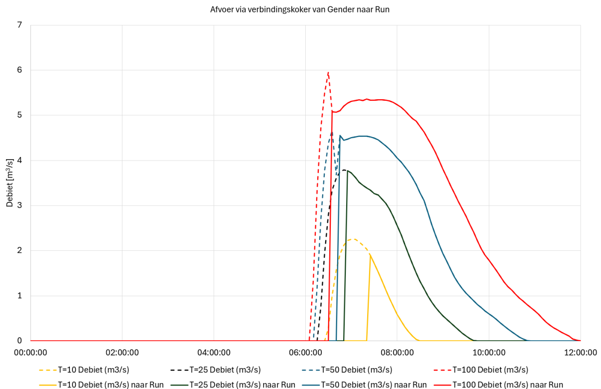
Figuur 2.2 Afvoer via verbinding van Gender naar Run voor buien met herhalingstijd T=25, T=50 en T=100. De gestippelde lijnen tonen het debiet dat via de overlaat de verbinding inloopt, de getrokken lijnen het debiet dat bij de uitstroomopening naar de Run uitstroom
