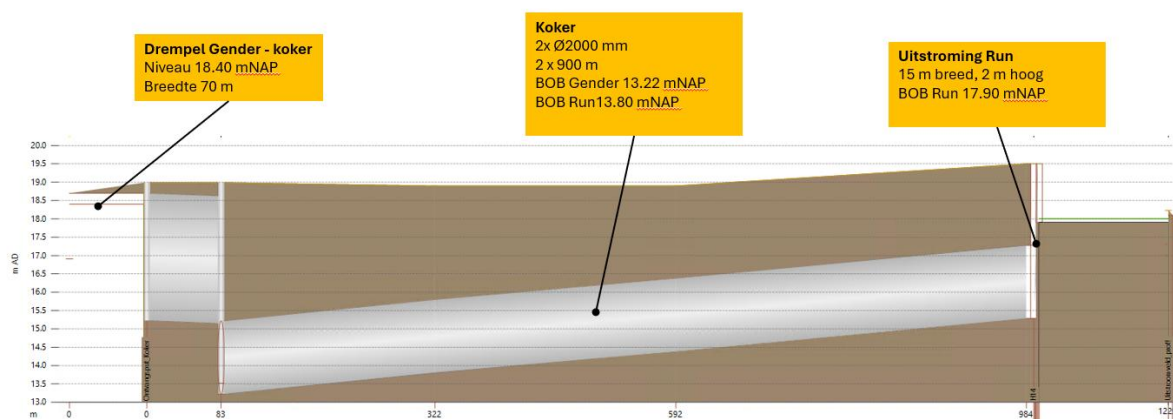
Figuur 2.1. Langsdoorsnede verbinding
