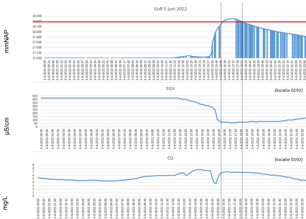
Figuur 2.3 Waterstand en waterkwaliteit in de Gender bij bui 5 juni 2022. De EGV (elektrische geleidbaarheid) daalt sterk tot een waarde rond de 50 \mu\text{S}/\text{cm} , hetgeen in de range ligt van afstromende neerslag. De zuurstofconcentratie stijgt eerst door de aanvoer van zuurstofrijk water uit verbeterd gescheiden stelsels en riooloverstorten, om daarna langzaam te dalen doordat het in het overgestorte water aanwezige BZV wordt omgezet.
