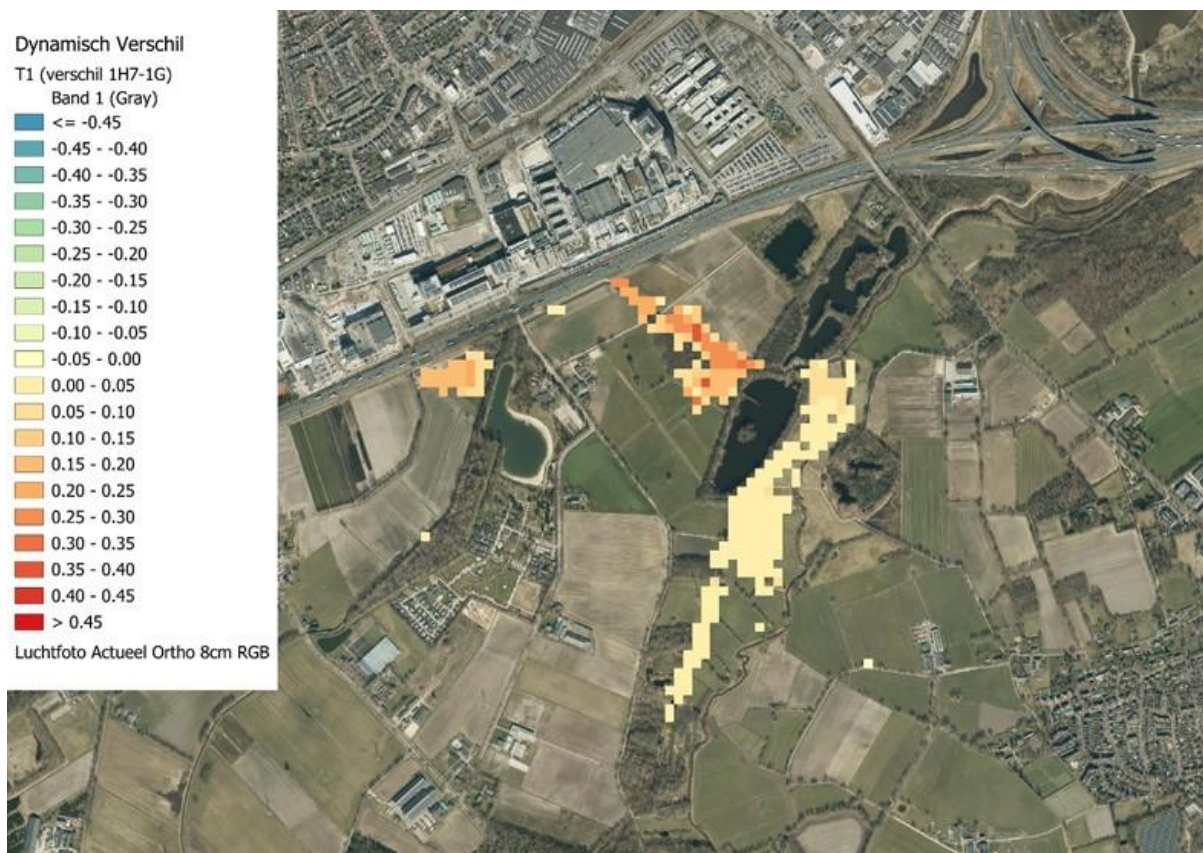
Figuur 22: Verschilkaart maximale waterdiepte bij T1 (beekherstel zonder inzet koppeling Gender-Run vergeleken met referentiesituatie). Groen-blauw betekent een afname van de waterdiepte en geel-rood een toename. Verschillen kleiner dan 2 centimeter zijn niet weergegeven
