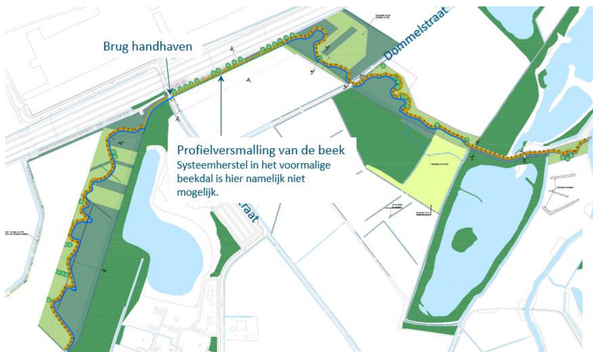
Figuur 33: Ontwerp beekherstel zonder koppeling Gender-Run (schetsontwerp)
