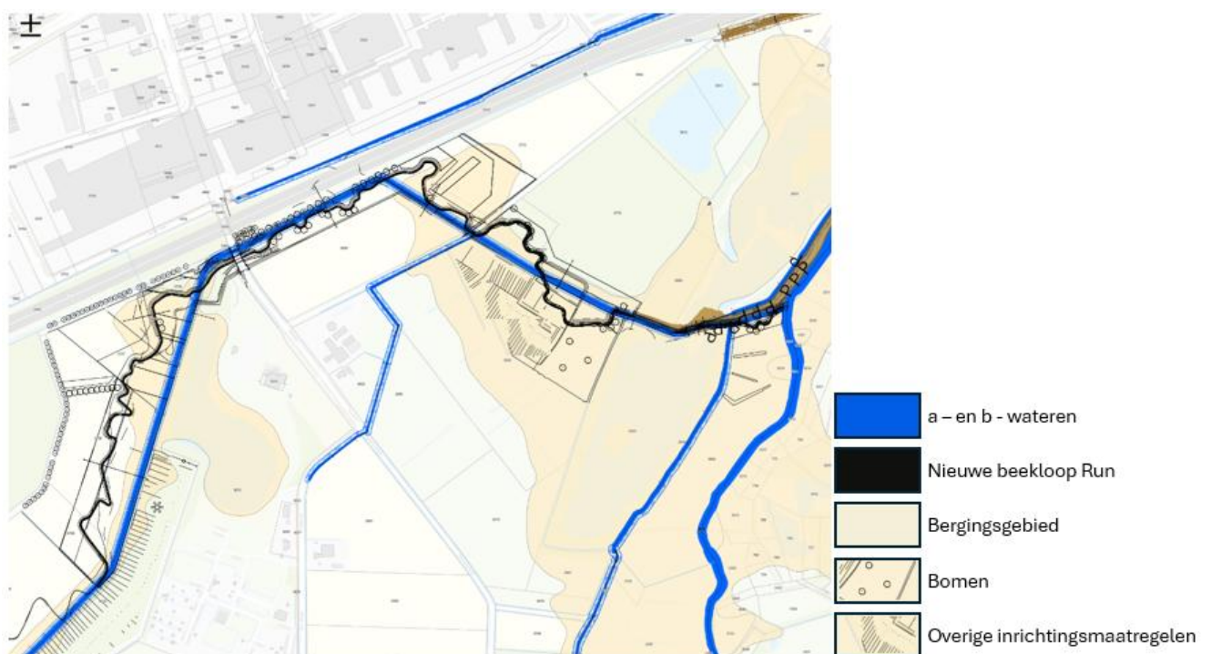
Figuur 19: Project Beekherstel Run Heers - Dommel op hoofdlijnen ten opzichte van de waterschapsverordening
