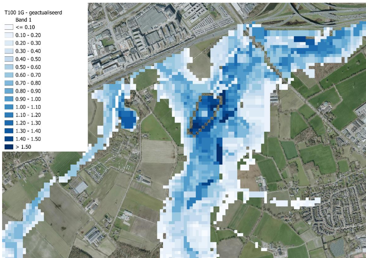
Figuur 26: Maximale waterdiepte bij T100 in referentiesituatie
