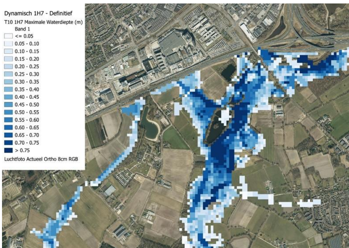
Figuur 24: Maximale waterdiepte bij T10 na realisatie beekherstel (zonder inzet koppeling Gender-Run)
