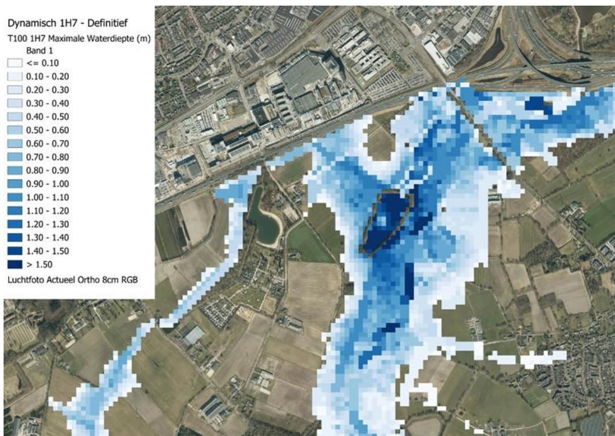
Figuur 27: Maximale waterdiepte bij T100 na realisatie beekherstel (zonder inzet koppeling Gender-Run)
