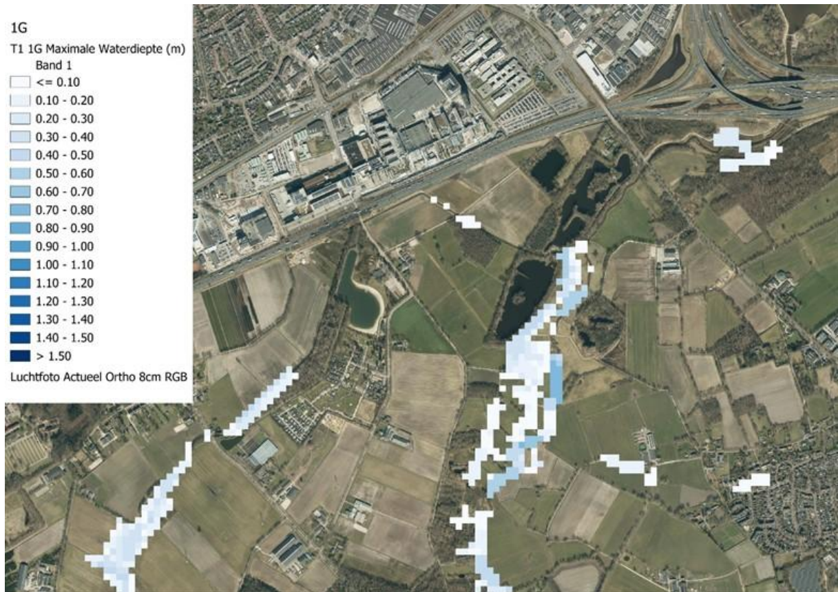
Figuur 20: Maximale waterdiepte T1 in referentiesituatie
