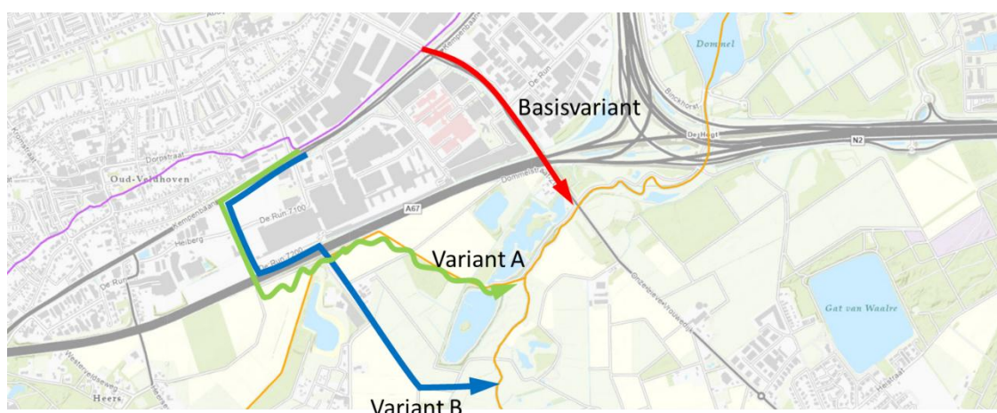
Figuur 31: Varianten oplossen waterproblematiek Gender
