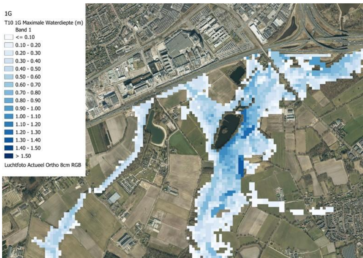
Figuur 23: Maximale waterdiepte bij T10 in referentiesituatie
