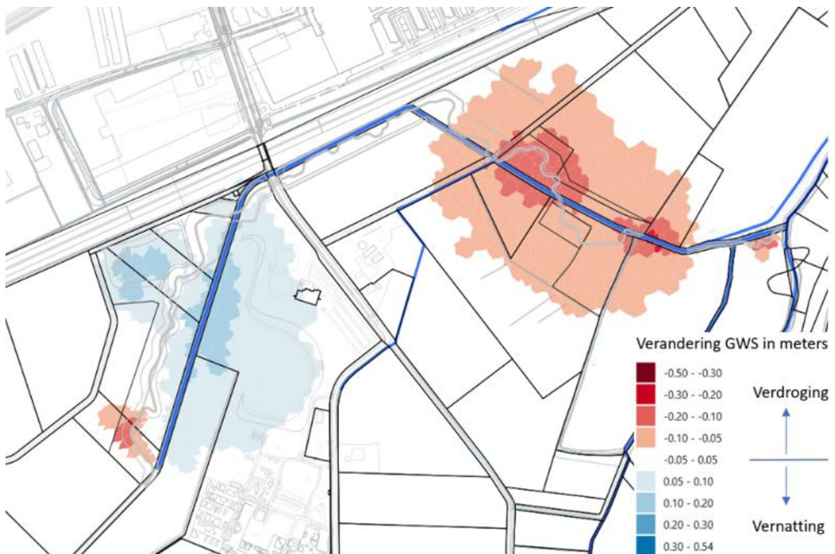
Figuur 30: Verandering in de Gemiddeld Laagste Grondwaterstand (GLG), gemiddelde zomersituatie
