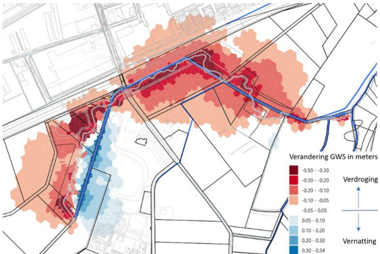
Figuur 29: Verandering in de Gemiddeld Hoogste Grondwaterstand (GHG), gemiddelde wintersituatie
