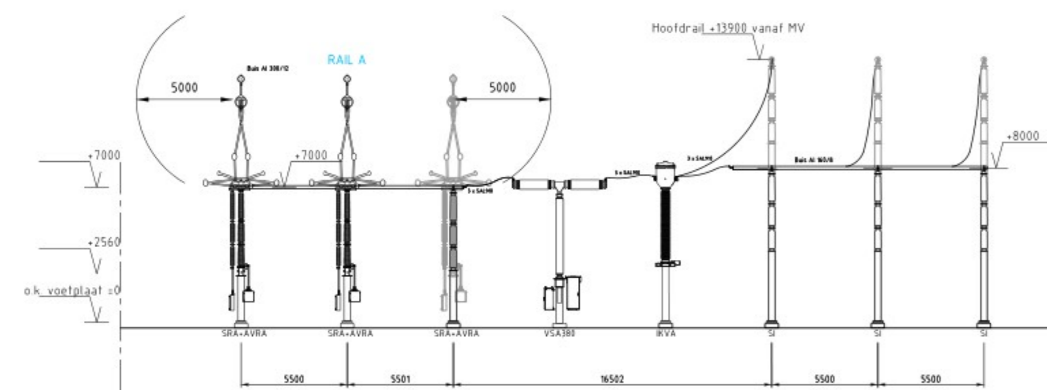
ZIJAANZICHT A-A 1:200
