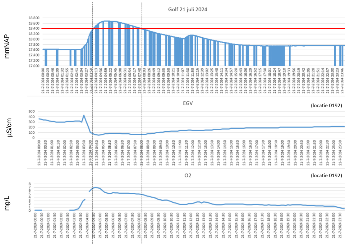
Figuur 2.5 Waterstand en waterkwaliteit in de Gender bij bui 21 juli 2024. De EGV (elektrische geleidbaarheid) daalt sterk tot een waarde tussen de 50-100 \mu\text{S/cm} , hetgeen in de range ligt van afstromende neerslag. De zuurstofconcentratie stijgt eerst fors tot 7 mg/l door de aanvoer van zuurstofrijk water uit verbeterd gescheiden stelsels en riooloverstorten, om daarna langzaam te dalen doordat het in het overgestorte water aanwezige BZV wordt omgezet.
