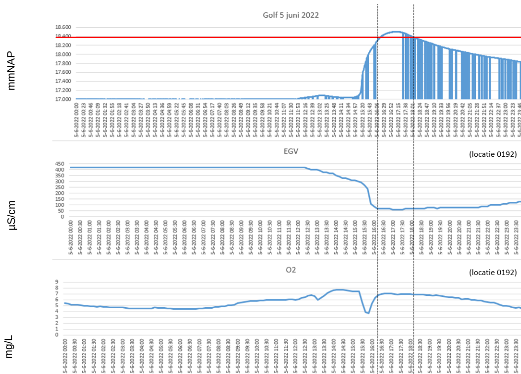
Figuur 2.4 Waterstand en waterkwaliteit in de Gender bij bui 5 juni 2022. De EGV (elektrische geleidbaarheid) daalt sterk tot een waarde rond de 50 \mu\text{S/cm} , hetgeen in de range ligt van afstromende neerslag. De zuurstofconcentratie stijgt eerst door de aanvoer van zuurstofrijk water uit verbeterd gescheiden stelsels en riooloverstorten, om daarna langzaam te dalen doordat het in het overgestorte water aanwezige BZV wordt omgezet.
