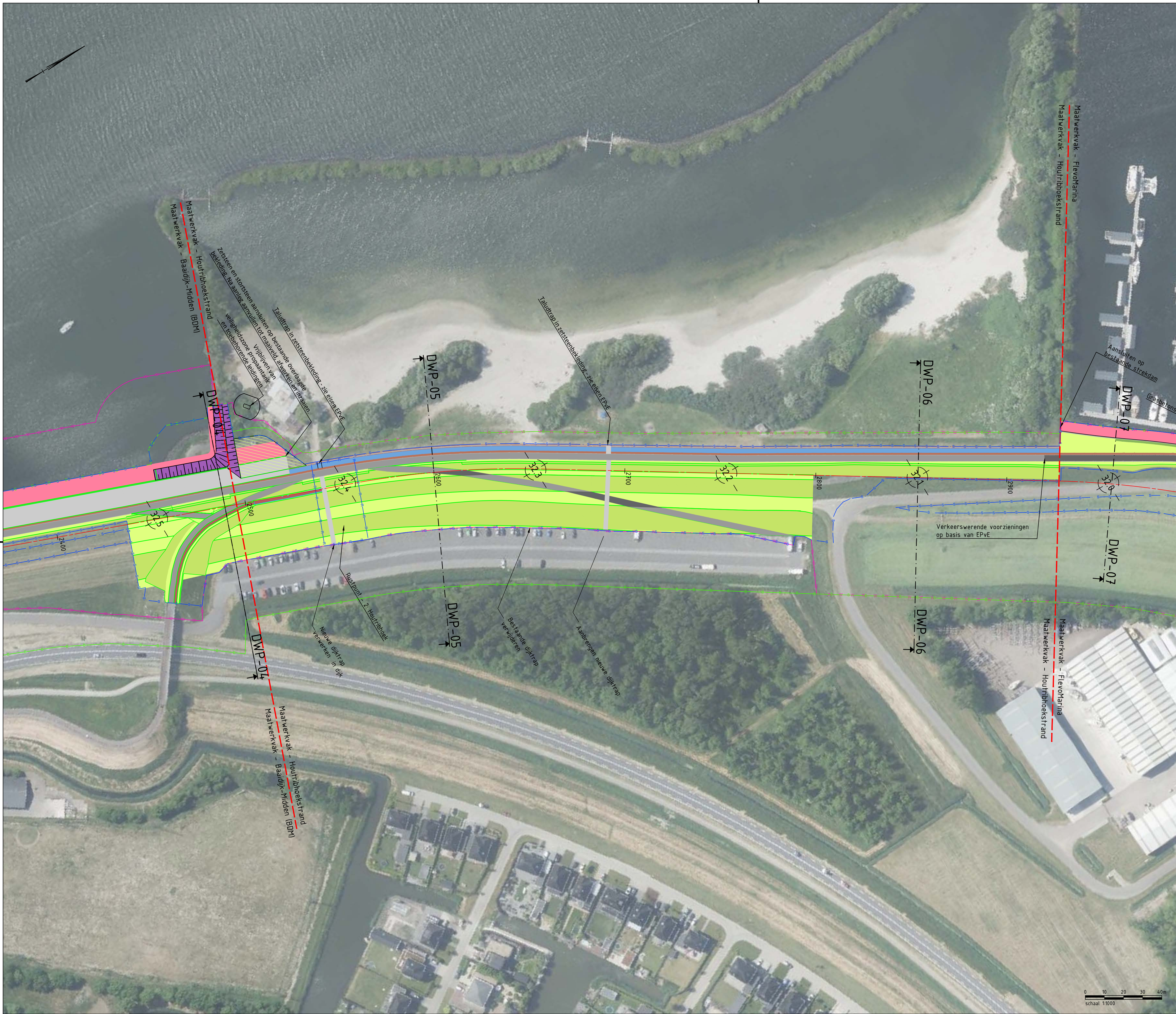
Overzicht - Detail Houtribhoekstrand SCHAAL 1 : 1000
