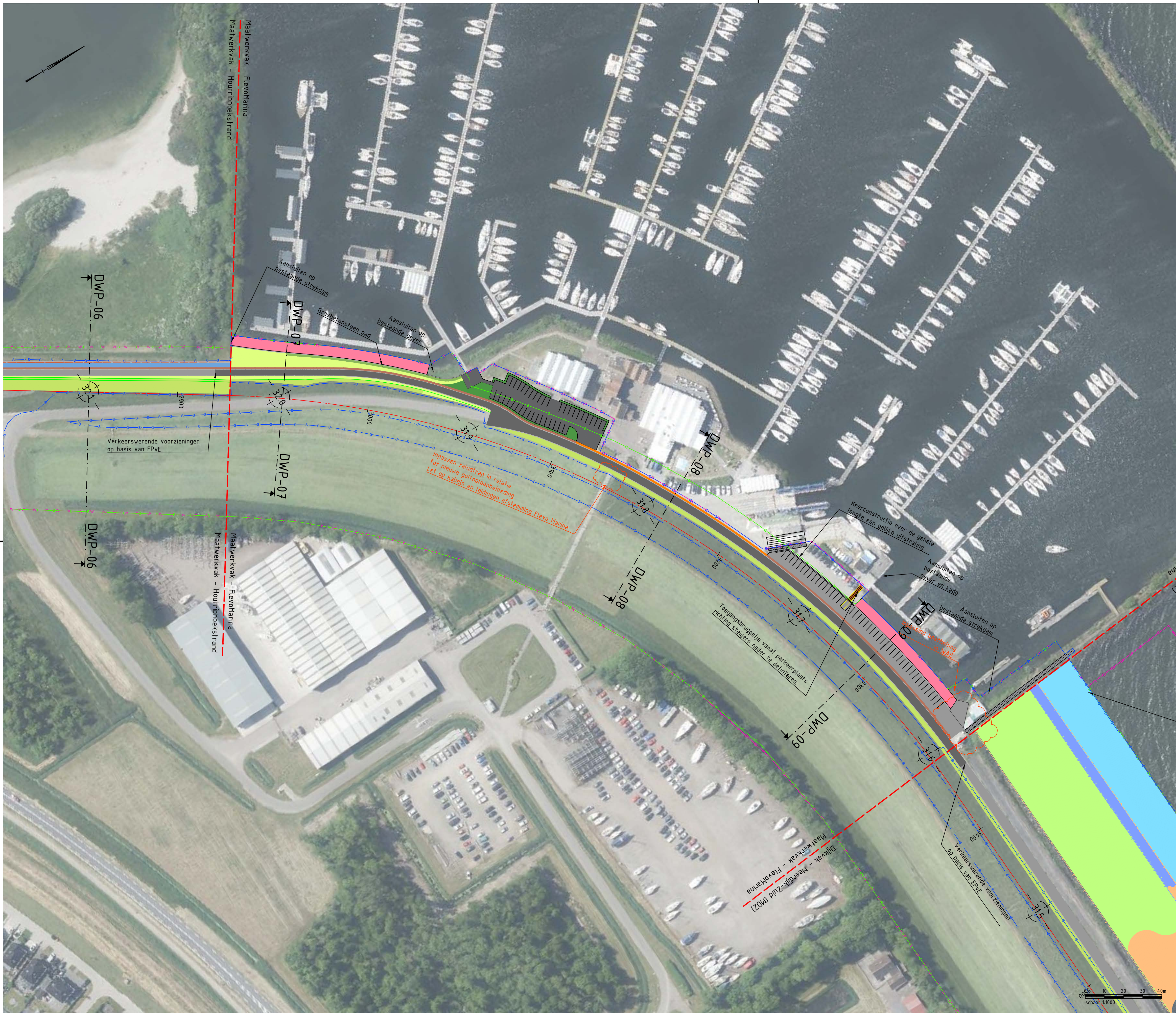
Overzicht - Detail Flevomarina SCHAAL 1 : 1000
