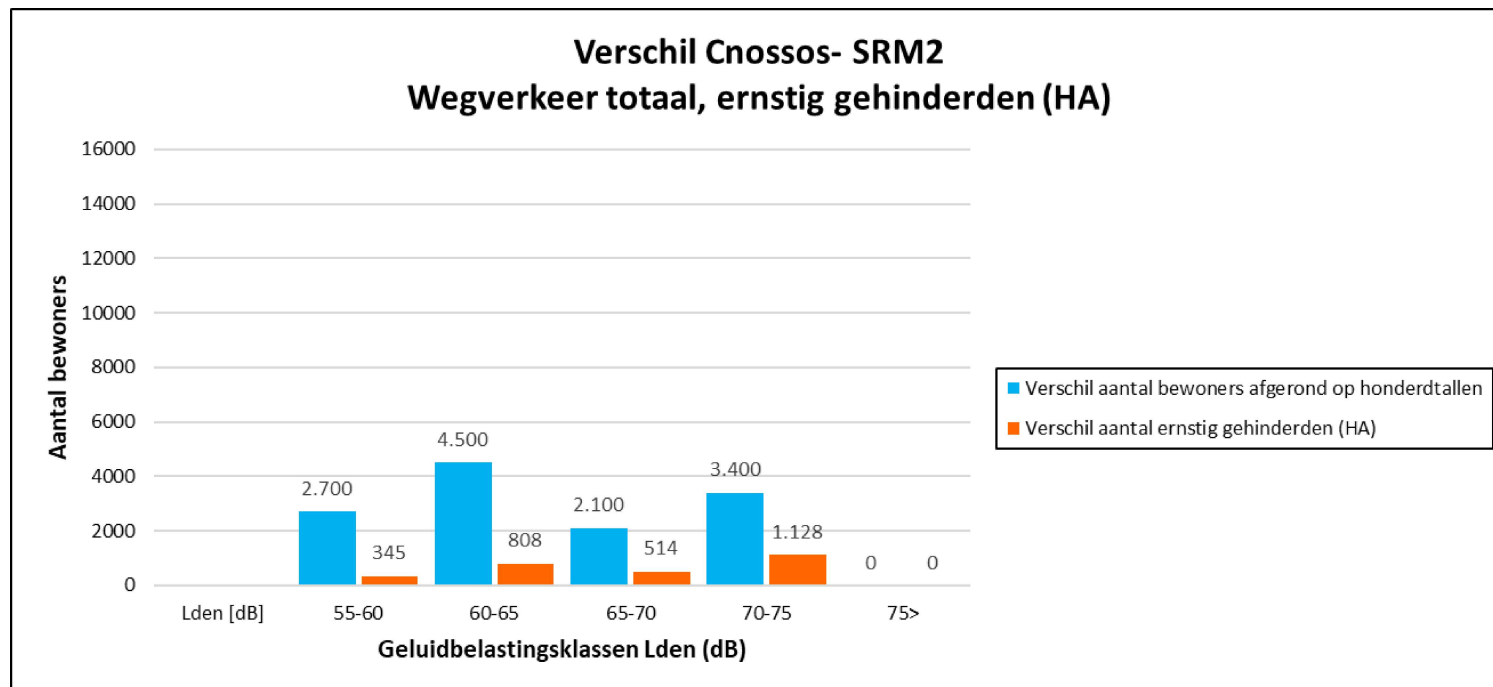
Figuur 19: verschil Cnossos en SRM2 gemeente Helmond 4e Tranche
