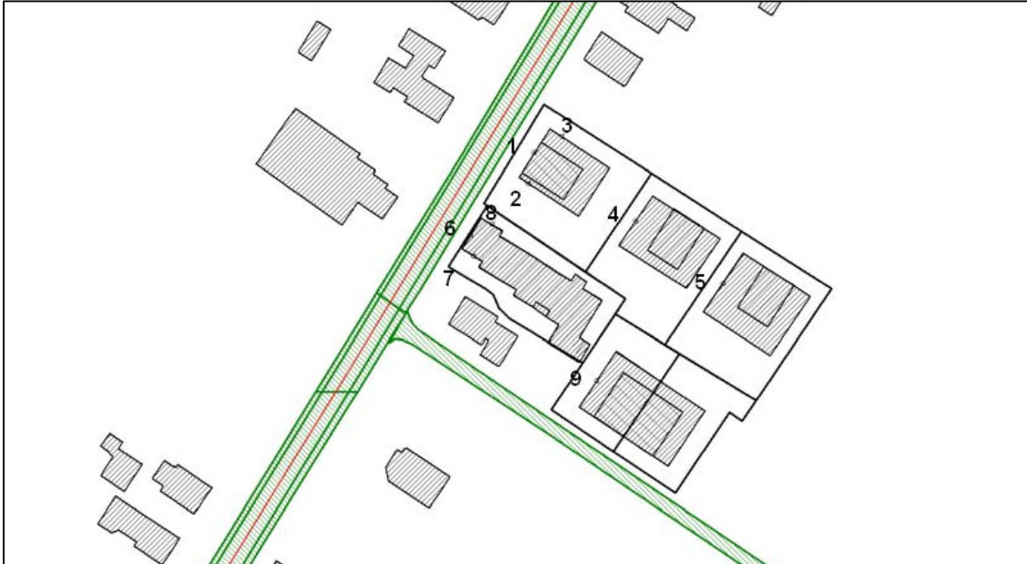
Figuur 2: Detail rekenmodel met rekenpunten
