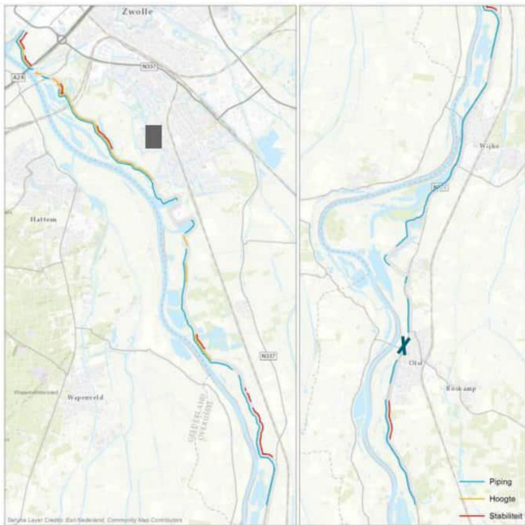
Figuur 2 Overzicht met aandachtspunten (faalmechanismen) voor de IJsseldijk (noordelijk deel links, zuidelijk deel rechts) (Bron: MER deel A)
