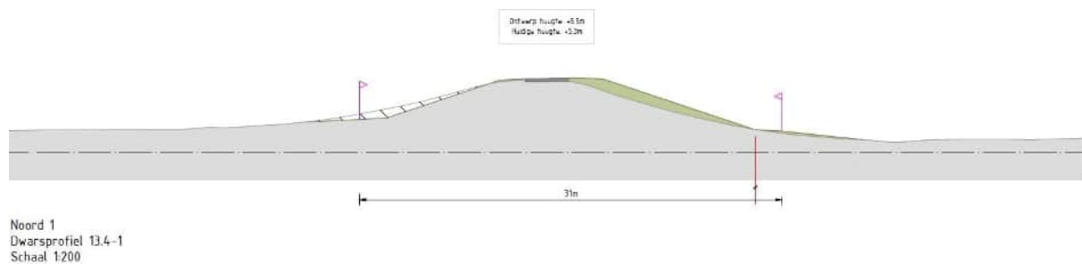
Afbeelding 5.36 Representatief dwarsprofiel deeltraject 13.4
