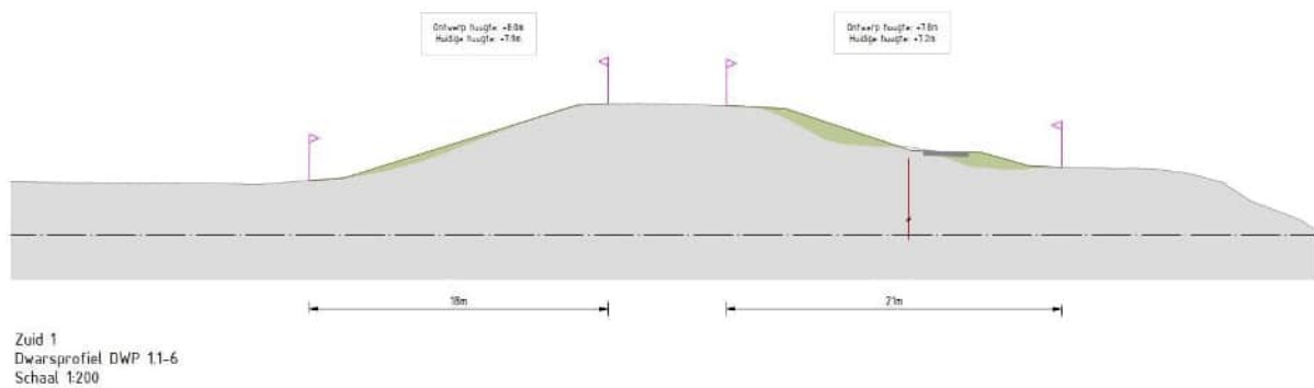
Afbeelding 5.2 Representatief dwarsprofiel deeltraject 1.1
