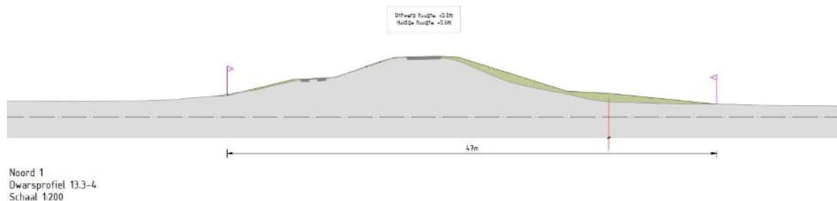
Afbeelding 5.35 Representatief dwarsprofiel deeltraject 13.3
