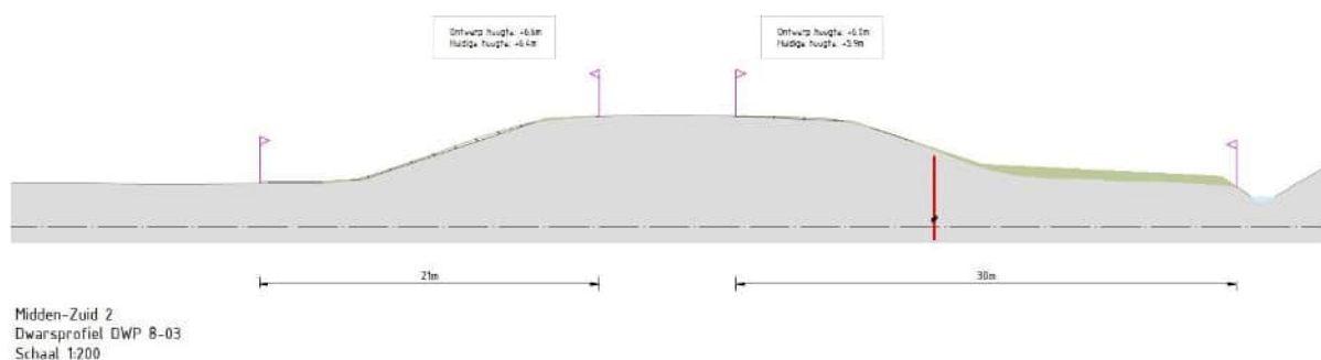
Afbeelding 5.16 Representatief dwarsprofiel deeltraject 8
