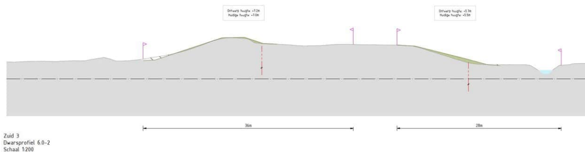
Afbeelding 5.11 Representatief dwarsprofiel deeltraject 6
