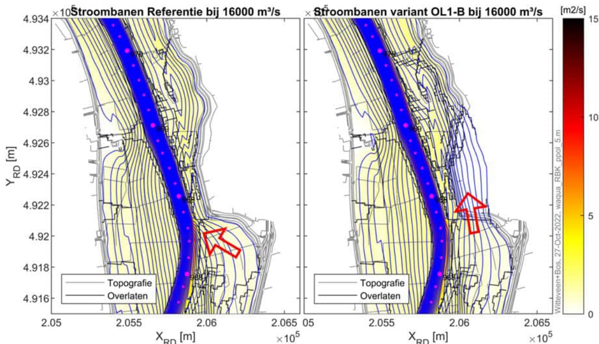
Afbeelding 9.4 Stroomlijnen voor referentie (links) en variant (rechts) bij een afvoer van 16.000 m³/s
