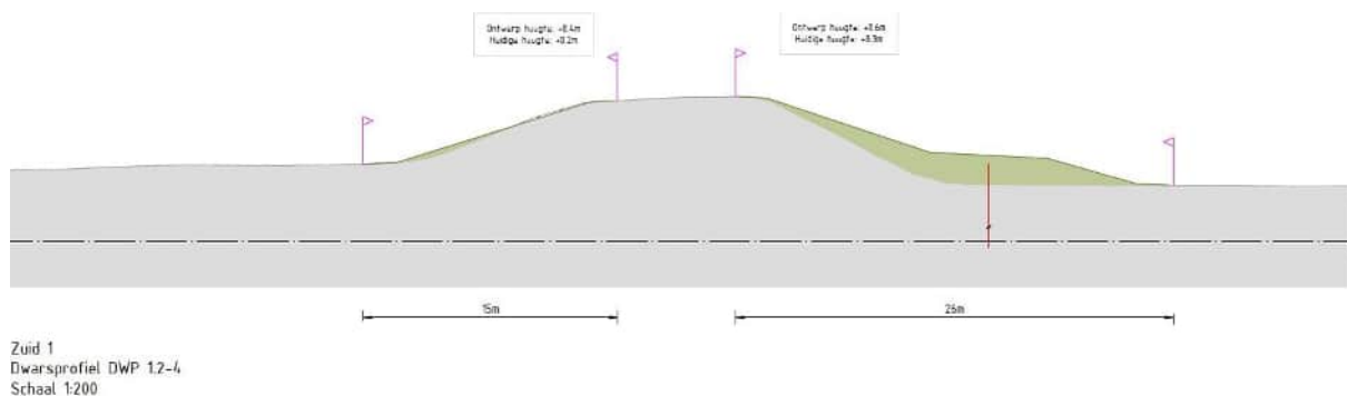
Afbeelding 5.3 Representatief dwarsprofiel deeltraject 1.2
