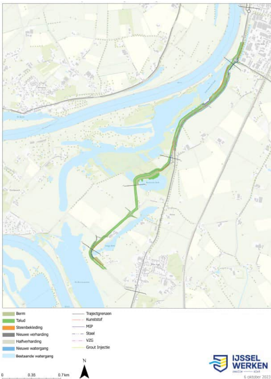
Afbeelding 5.12 Dijkversterkingsontwerp dijkmodule Zuid 3
