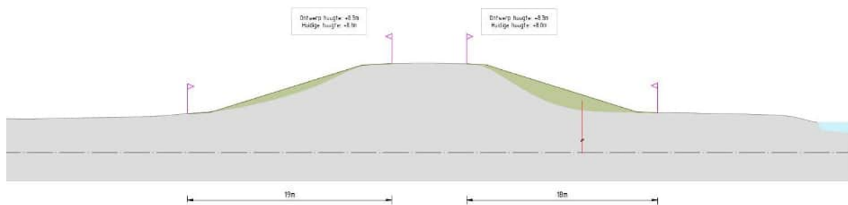
Afbeelding 5.4 Representatief dwarsprofiel deeltraject 2
