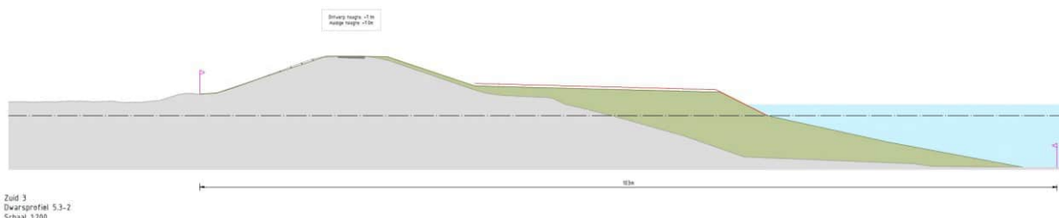
Afbeelding 5.10 Representatief dwarsprofiel deeltraject 5.3
