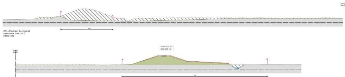
Afbeelding 5.17 Representatief dwarsprofiel deeltraject 9a
