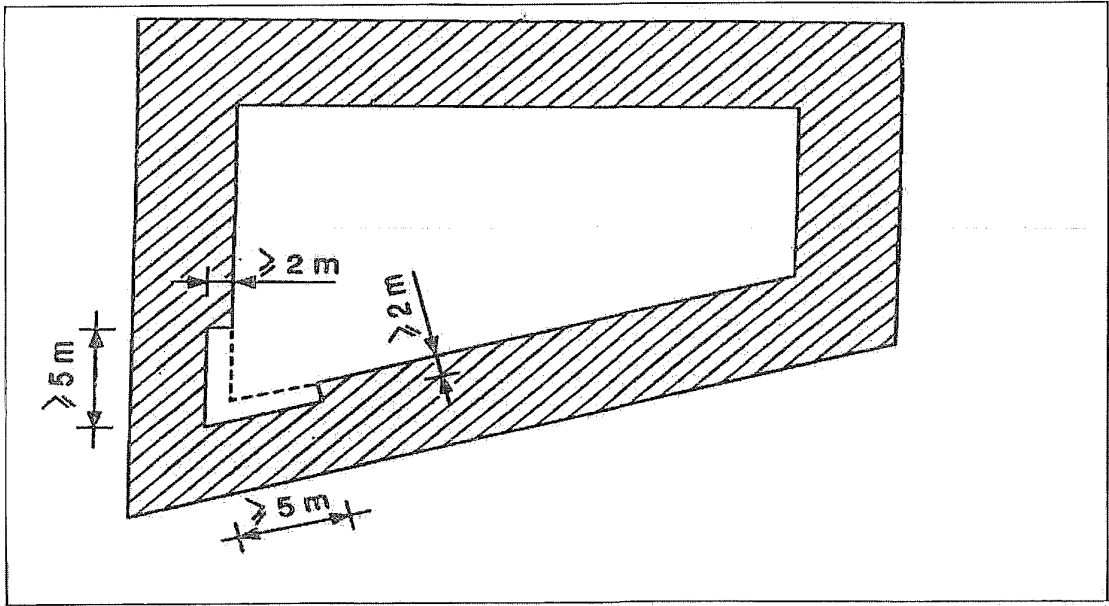
Figuur 10 Ligging van de achtergevelrooilijn (artikel 2.5.11, eerste lid, onder e)
