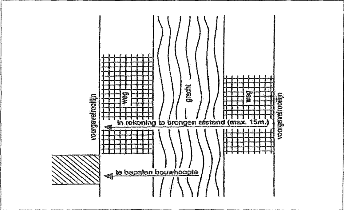
Figuur 15 Bouwhoogte in de voorgevelrooilijn (artikelen 2.5.20, derde lid, eerste alinea)
