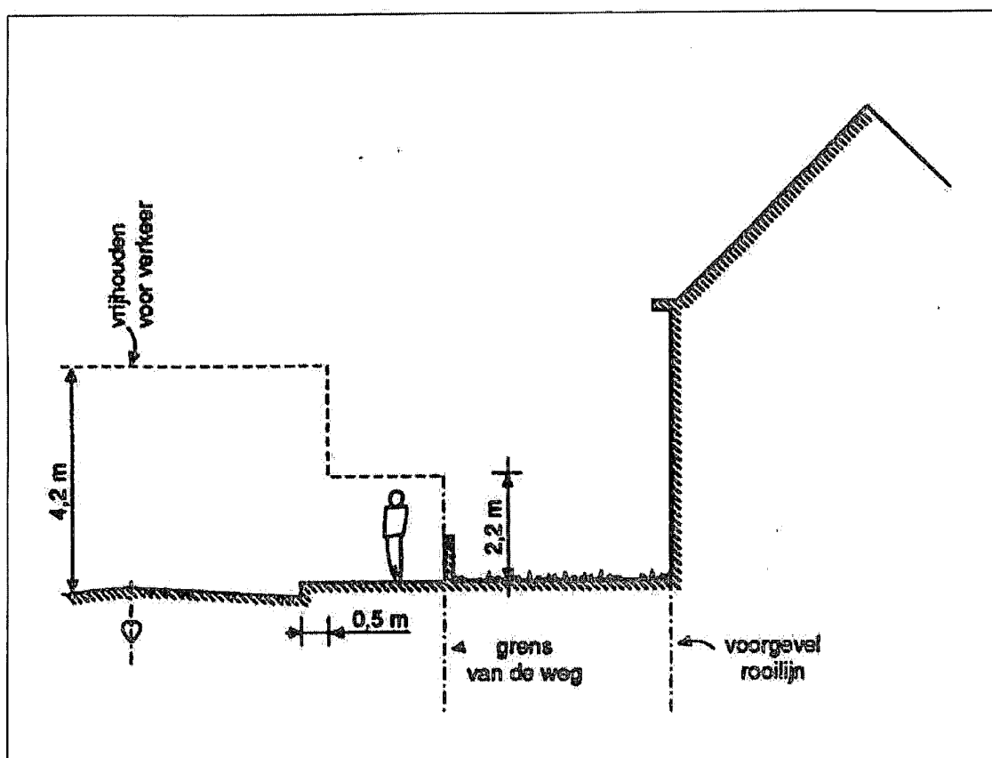
Figuur 1 Voor verkeer vrij te houden hoogten (artikel 2.5.11, eerste lid, onder c)
