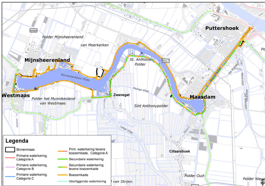
Figuur 4: Waterkeringen
