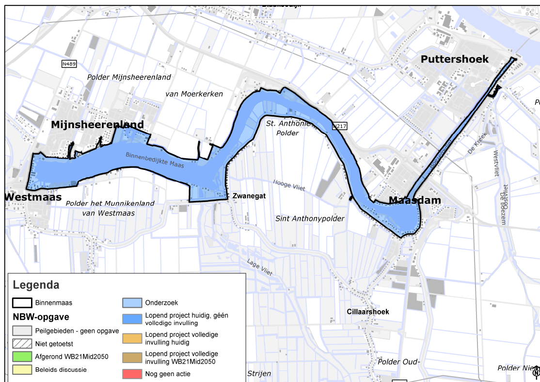
Figuur 8: Wateropgave
