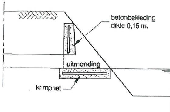
Dwarsdoorsnede A-A
