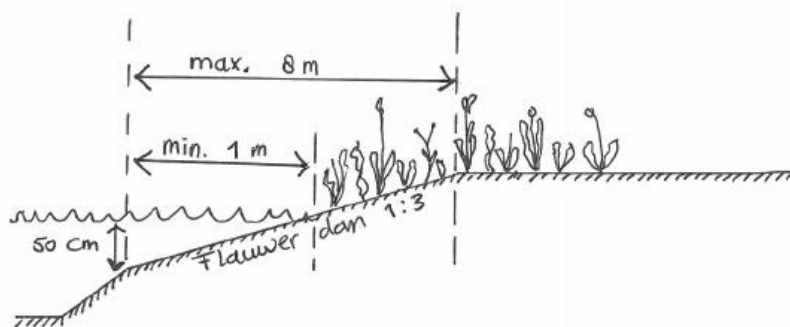
Principetekening algemene regel nr 26: ontgraving oever
