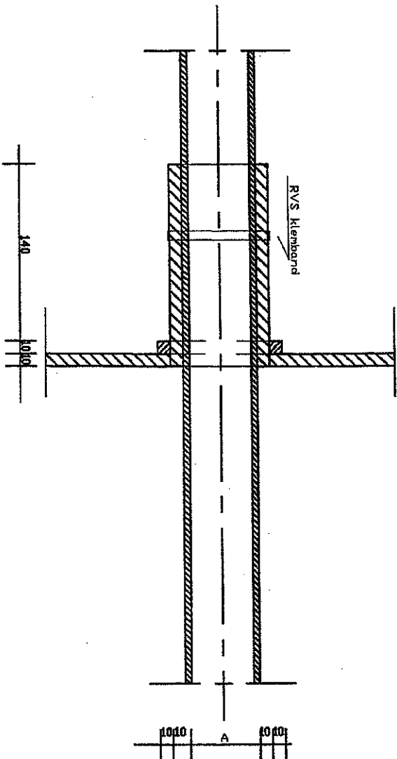
ZIJAAANZICHT / LANGSDOORSNEDE
