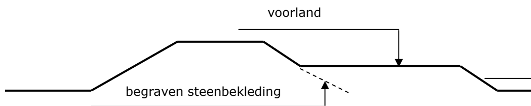
Figuur 1 Schematisatie kering met voorland en begraven steenbekleding
