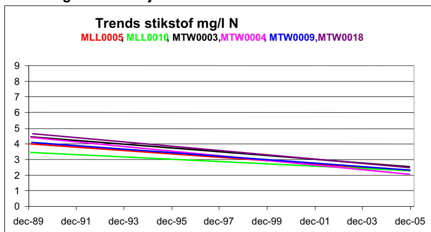
afbeelding 2.5. Trendlijnen stikstof Tielerwaard 1990-2005
