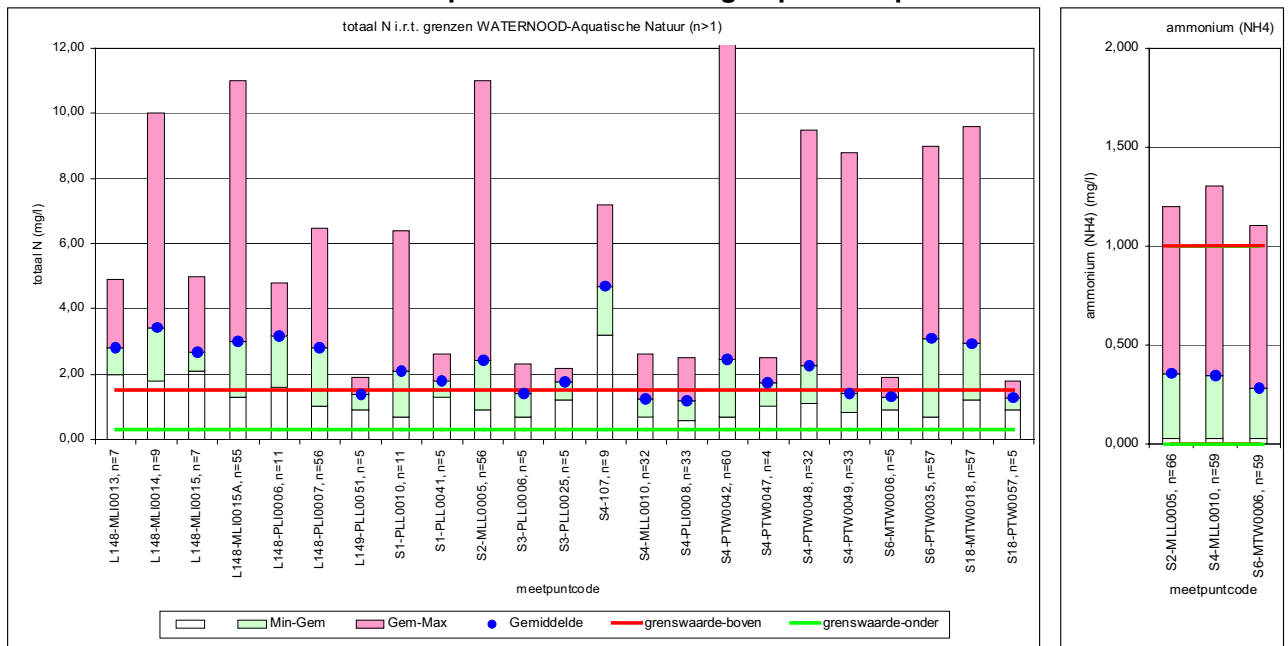
afbeelding 7.2. Totaal N en ammonium (NH 4 ) in vergelijking met de grenswaarden, zoals gedefinieerd in de module aquatische natuur van Waterlood: op de x-as staan de SED-watervallen met meetpunt en aantal metingen per meetpunt
