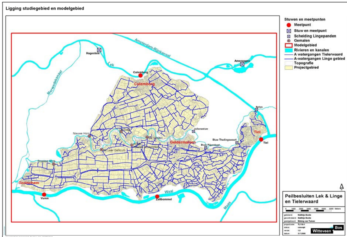
afbeelding 2.1. Ligging Lek & Linge en Tielertaard
