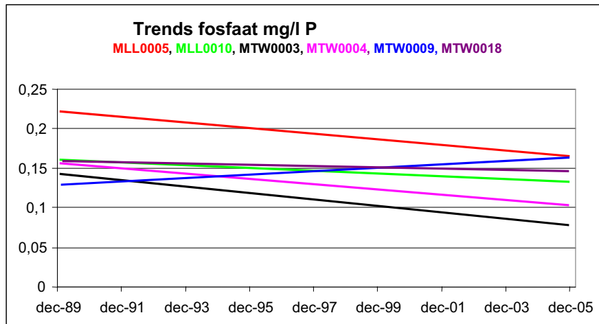
afbeelding 2.6. Trendlijnen fosfaat Tielerswaard 1990-2005
