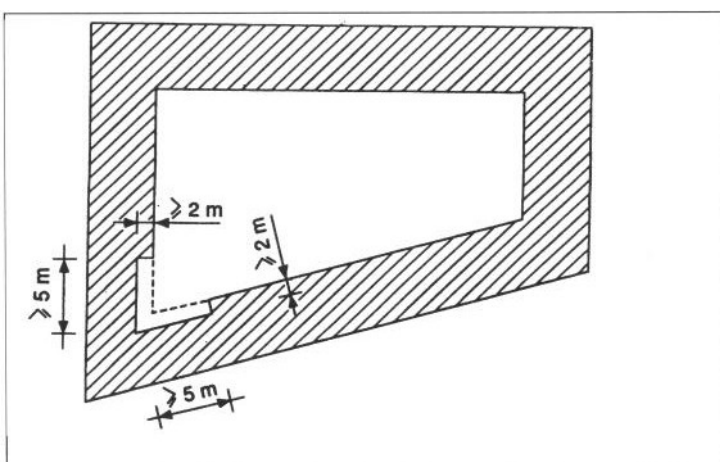
Figuur 11 Teruglegging met het oog op de toetreding van het daglicht van de achtergevelrooilijn die een scherpe hoek met elkaar vormen (ingevolge artikel 2.5.11 lid 2)
