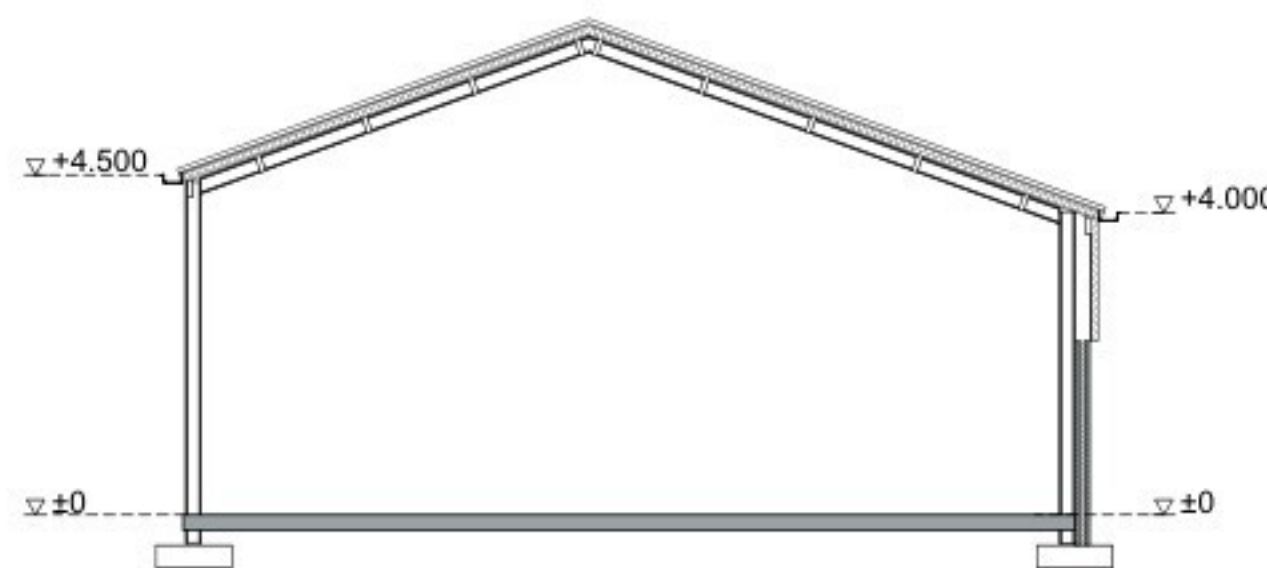
Doorsnede gebouw D
