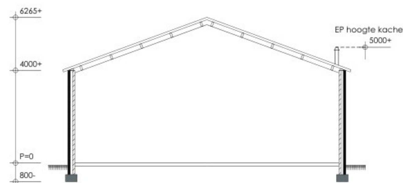
Doorsnede gebouw C
