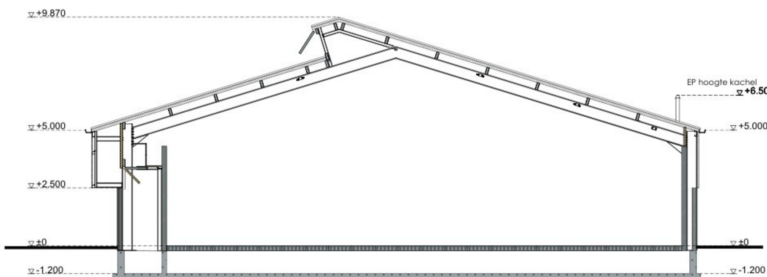
Doorsnede gebouw A en B
