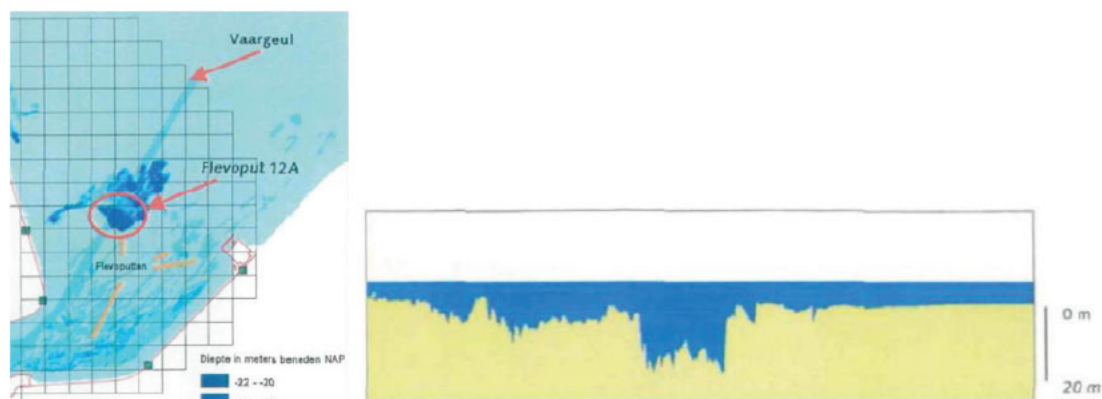
Figuur 5.1 Links: ligging van Flevoput 12A, rechts: dwarsdoorsnede Flevoput 12A en omgeving. Links is noordwest en rechts is zuidoost (Van Rijn et al. , 2004), aangeduide vaargeul betreft Vaargeul Amsterdam Lemmer (VAL)
