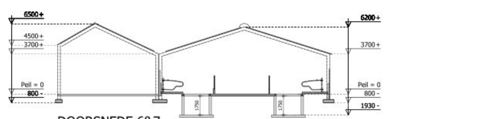
DOORSNEDE 6&7
