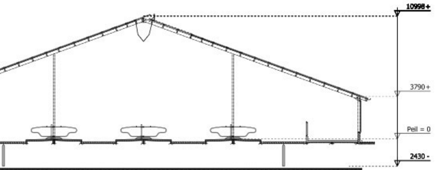
DOORSNEDE 8
