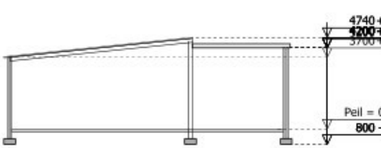
DOORSNEDE 5
