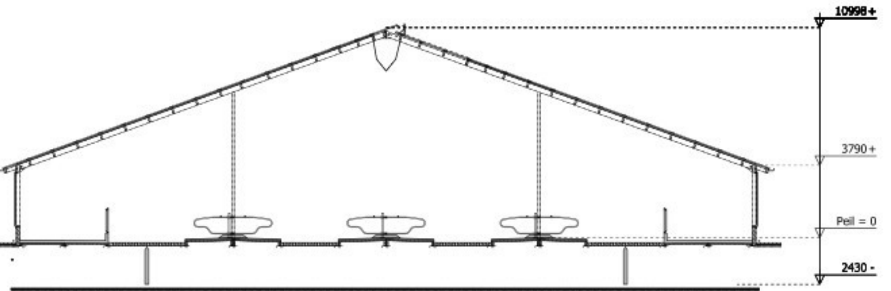
DOORSNEDE 9
