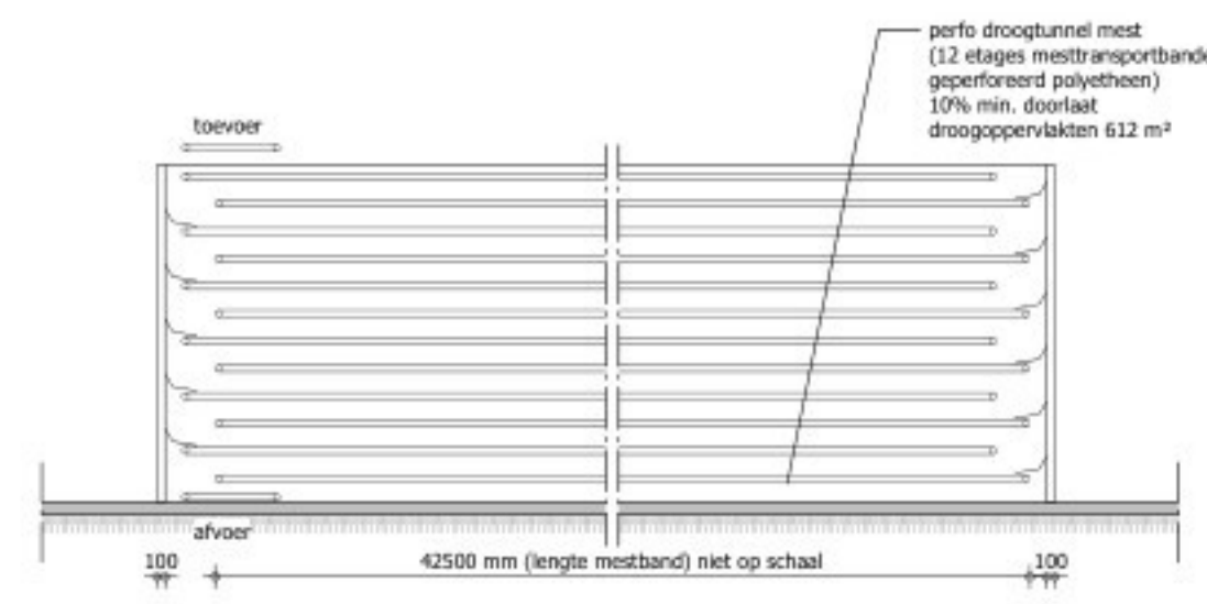
Langtedoorsnede droogtunnel
