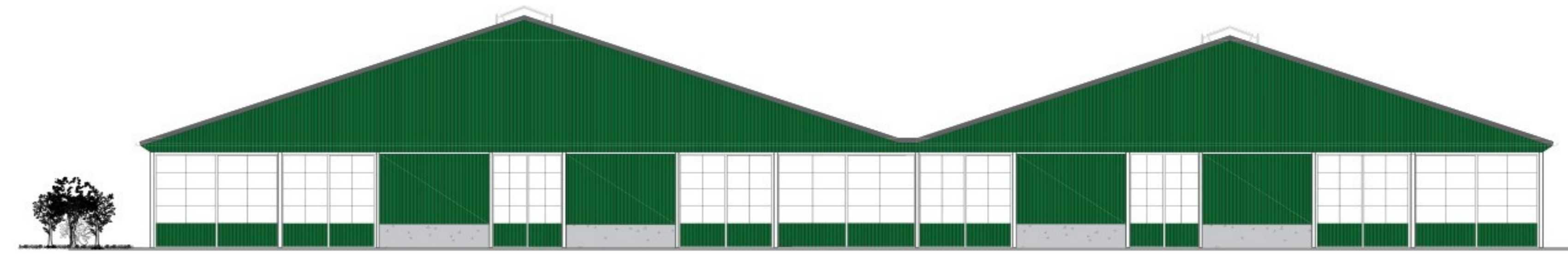
aanzicht oost
