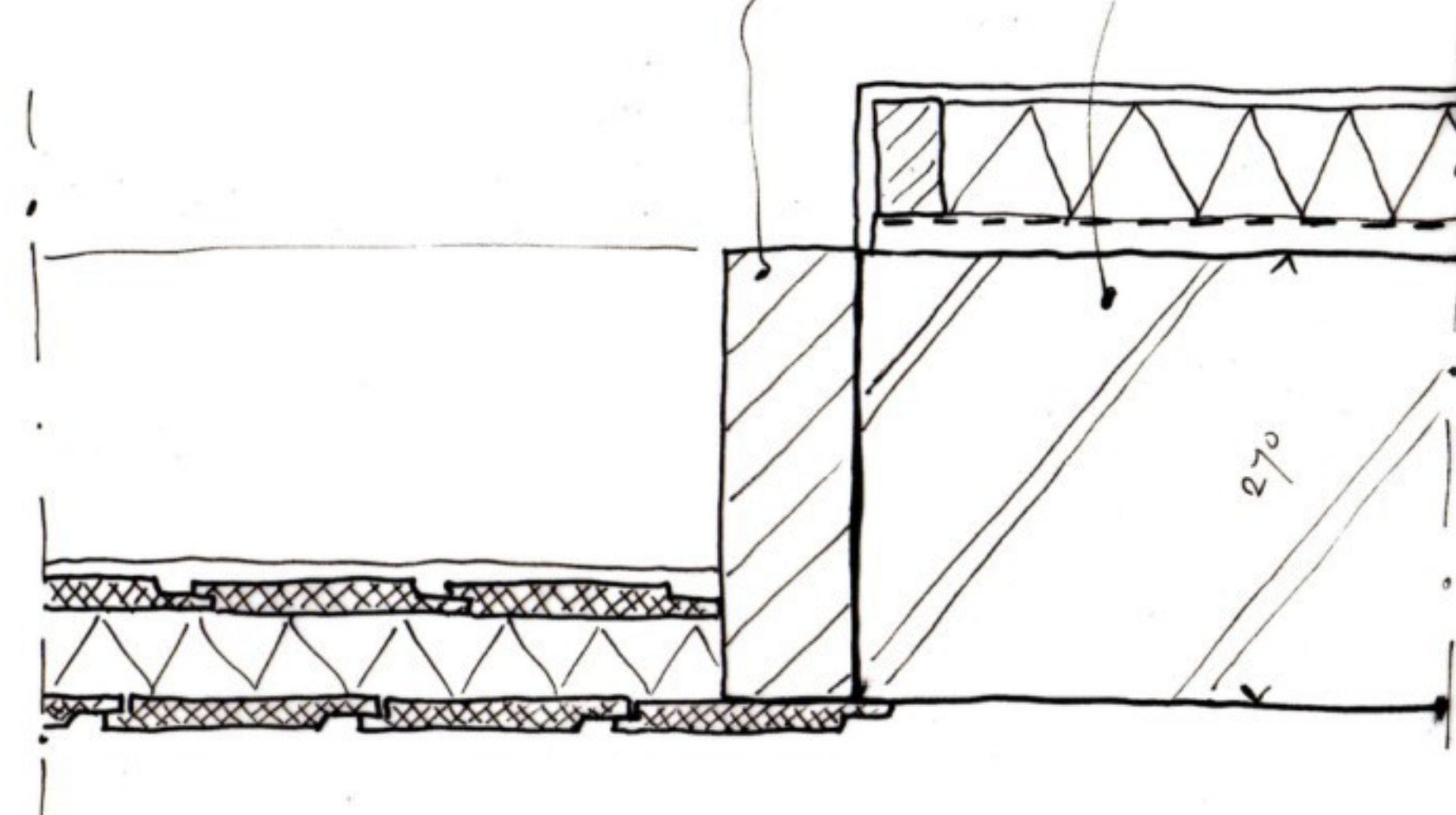
principe stalen pui
