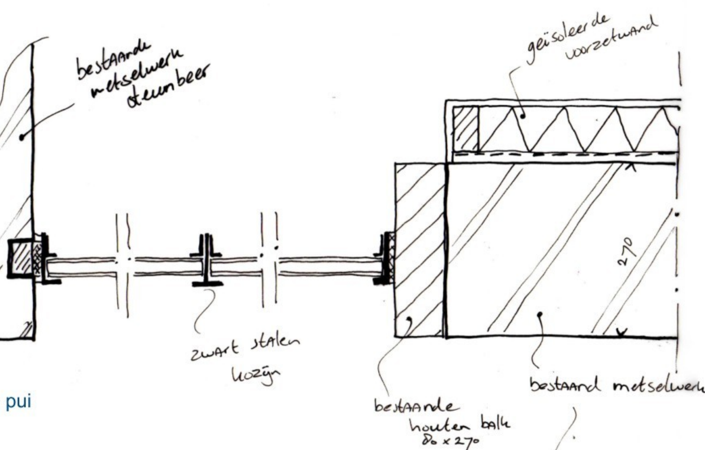
principe stalen pui
