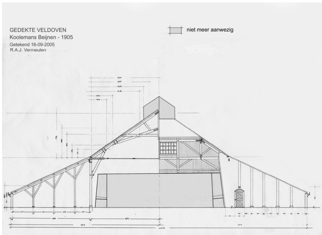
Reconstructietekening 2005
