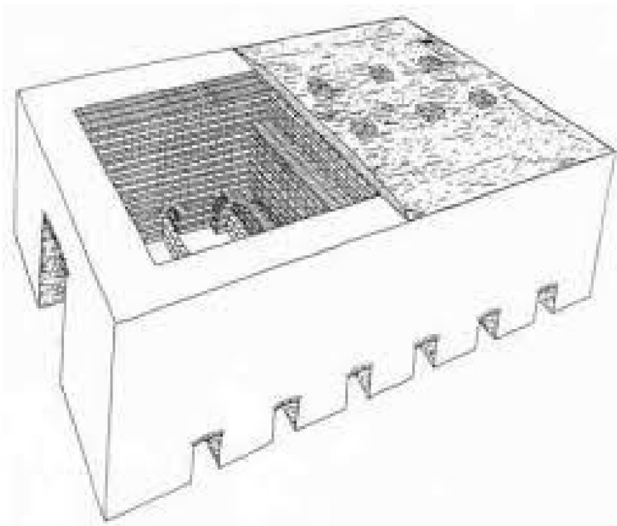
Principe opbouw Hollandse veldoven
