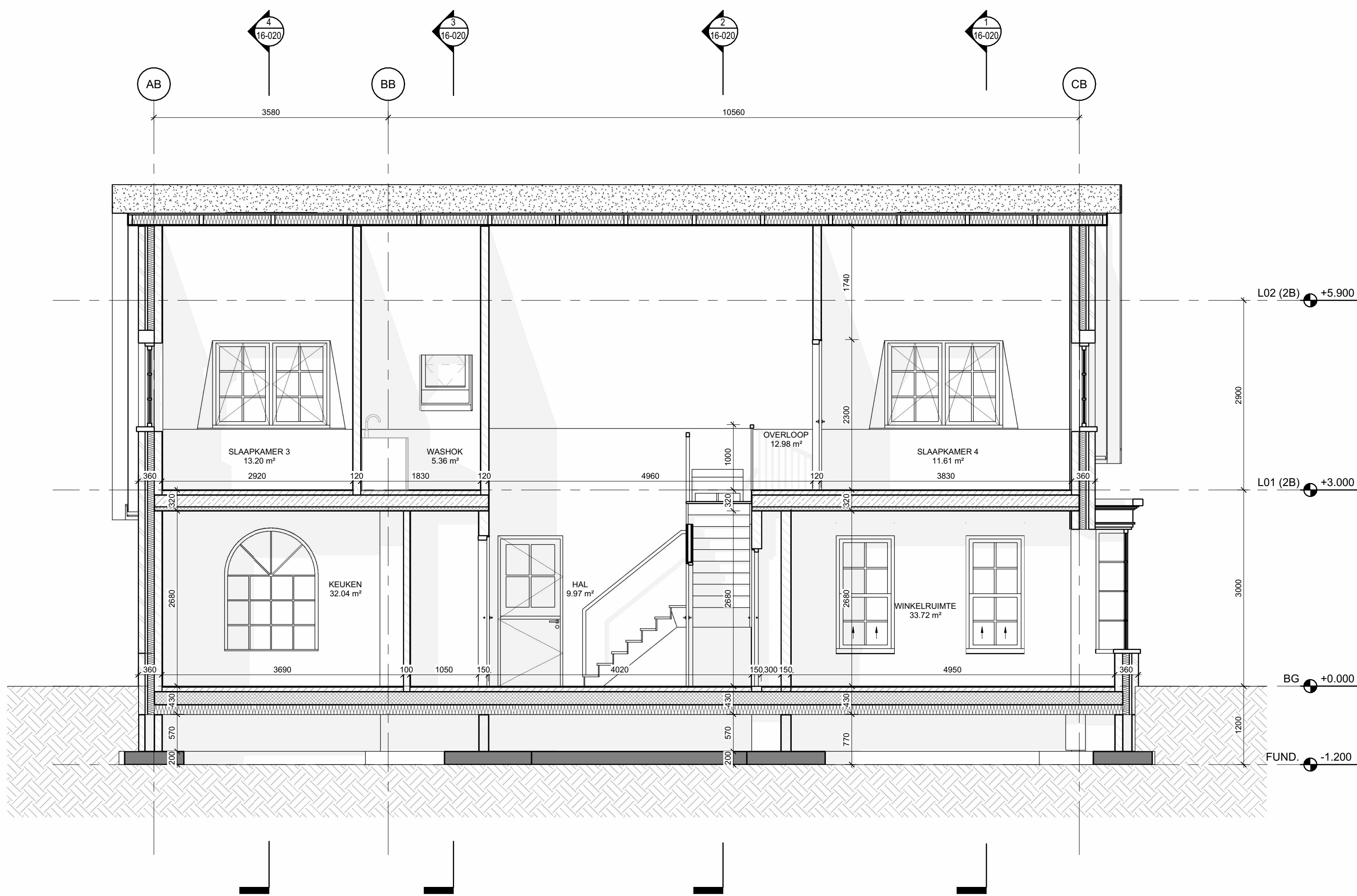
2B - LANGSDOORSNEDE A SCALE: 1 : 50
