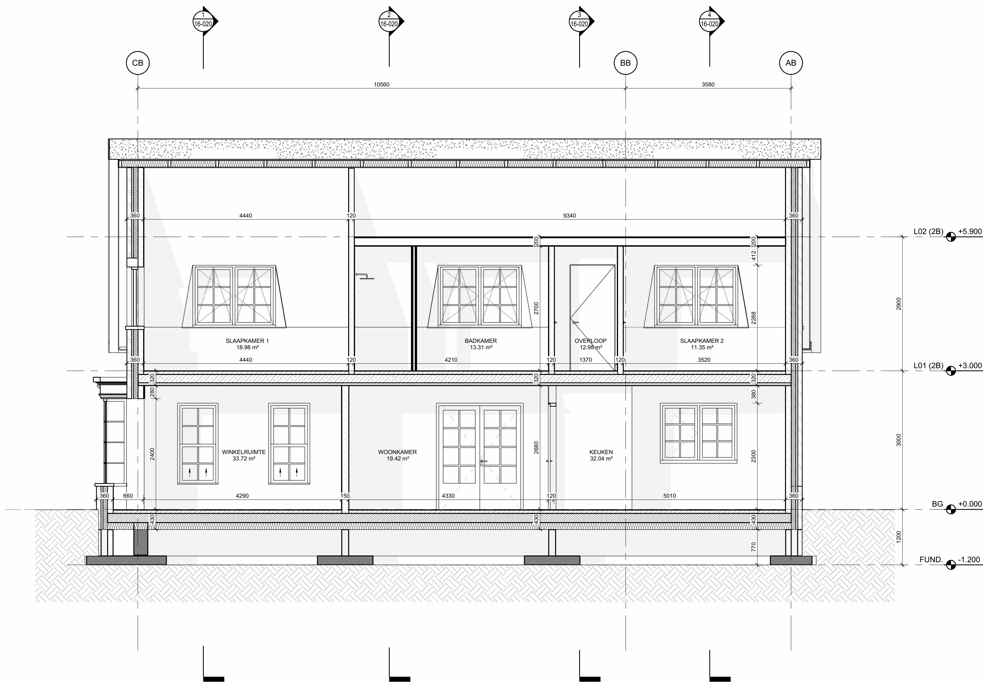
2B - LANGSDOORSNEDE B SCALE: 1 : 50
