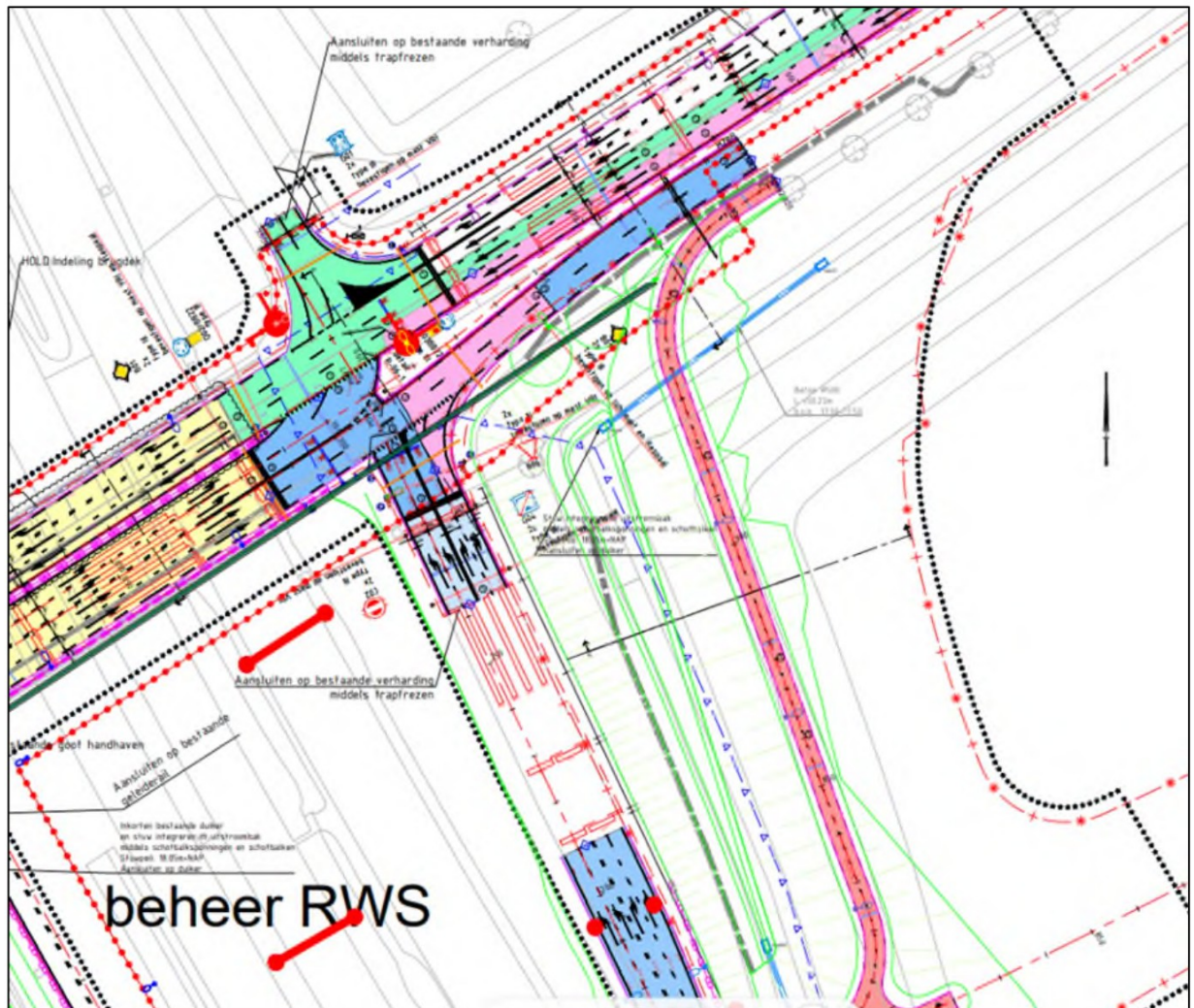
Figuur 2-17: Afwatering oostelijk deel A2/N2 (Bron: Uitvoeringsontwerp A. Fokkerweg, gemeente Eindhoven, d.d. 10-05-2019).
