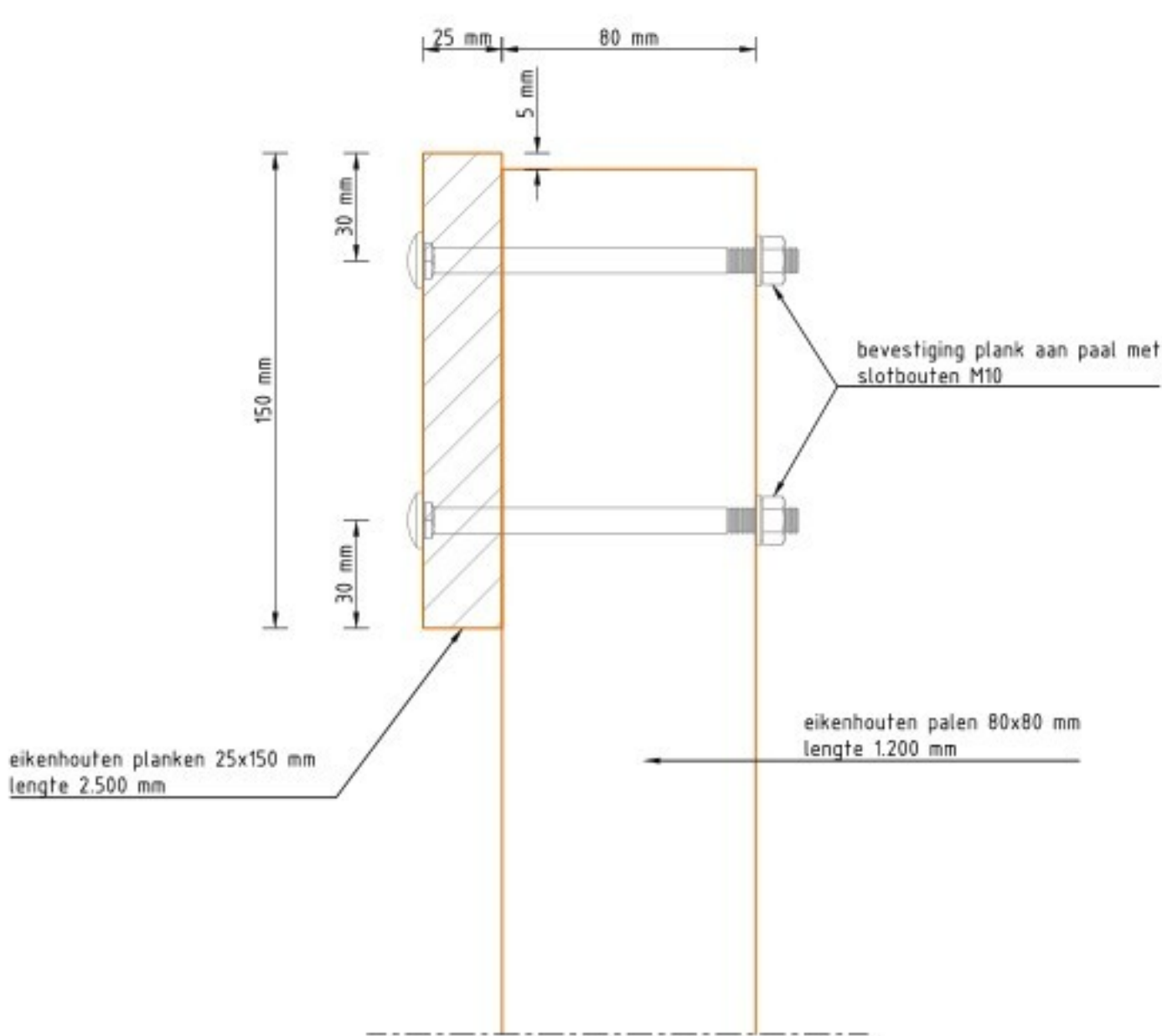
Detail 01 schaal 1:2
