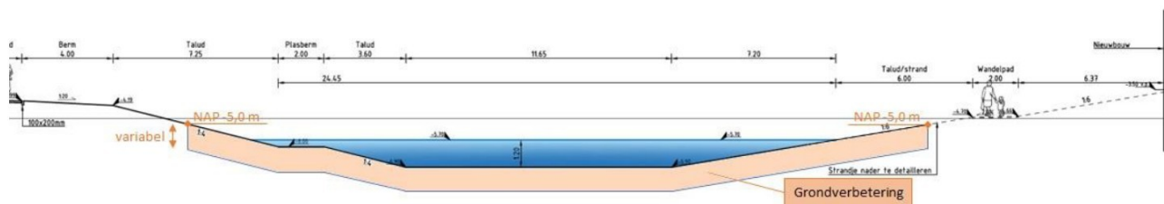
Figuur 11 Principe dwarsprofiel vak G01 met grondverbetering
