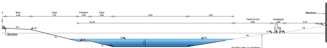
Figuur 4 Principe dwarspofiel vak G01
