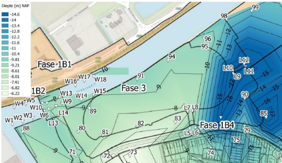
Figuur 6 Diepte bovenkant eerste zandlaag Zeelandse Oostvaardersdijk
