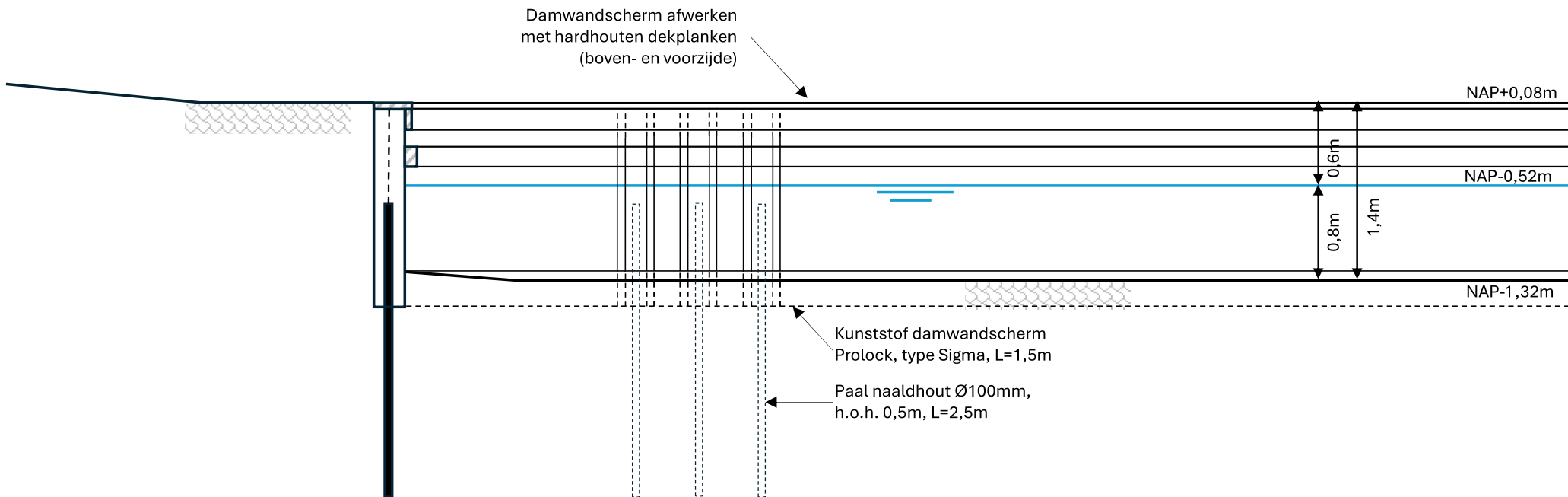
AANZICHT BESCHOEIING
