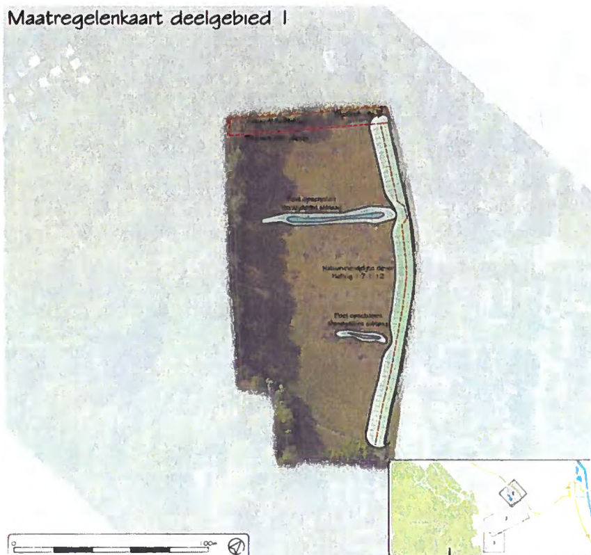
Figuur 4. Nieuwe inrichting van deelgebied 1 met als beoogde maatregelen: hekwerk verwijderen en opnieuw aanbrengen (rode stippellijn); twee poelen opschonen (licht- en donkerder blauwe vlak); en natuurvriendelijke oever aanleggen (lichtgroen gestreept vlak).
