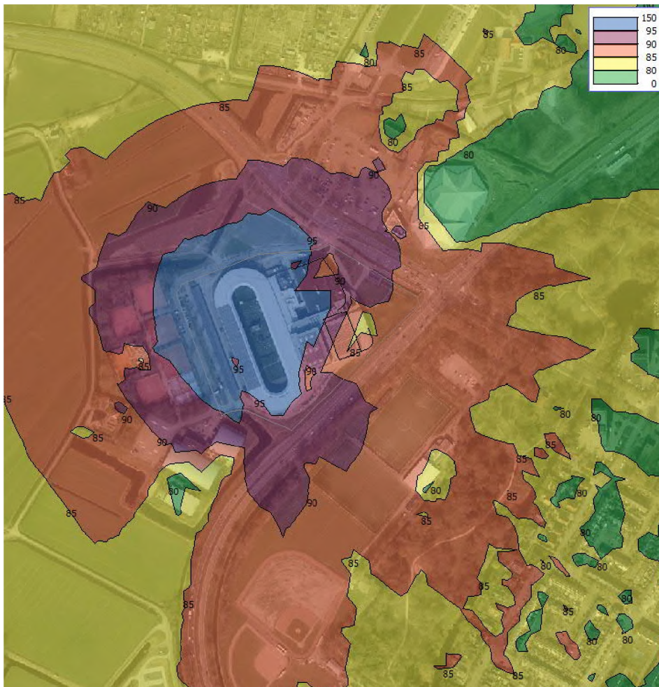
Figuur 5 Geluidscontouren incidentele bedrijfssituatie (met noord opstelling)
