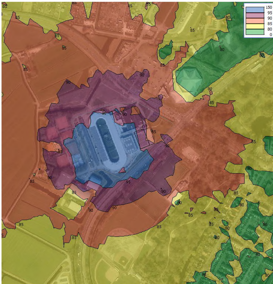
Figuur 6 Geluidscontouren incidentele bedrijfssituatie (met zuid opstelling)
