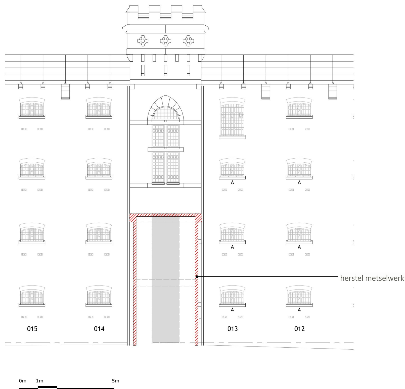
Toren zuid - bestaande situatie
