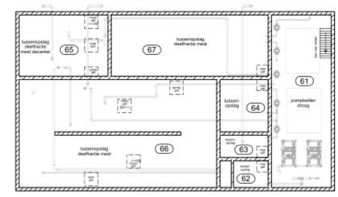
Kelder Geniaalconcept
