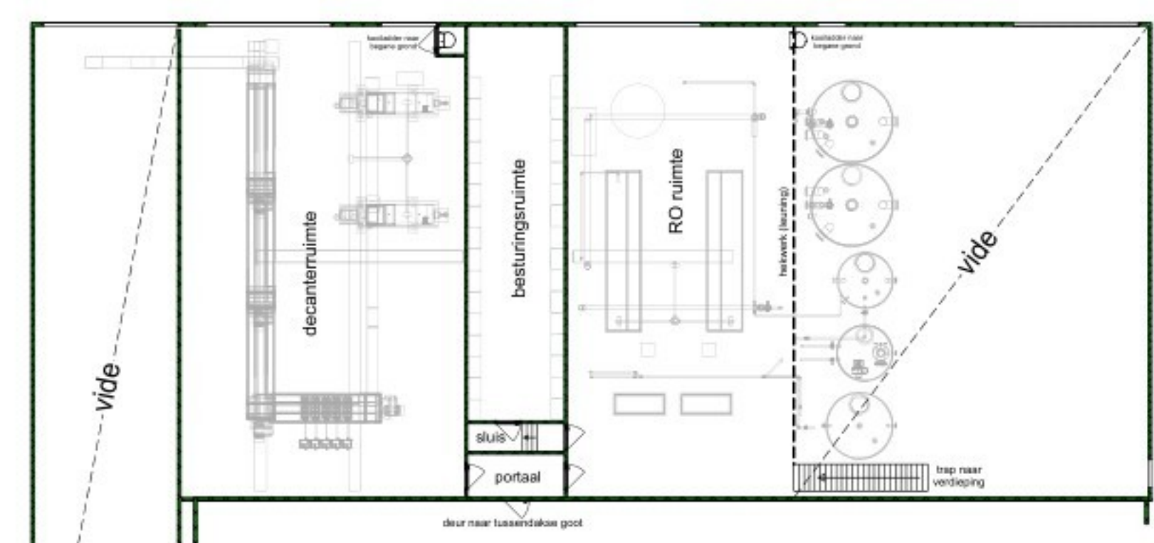
Verdieping Geniaalconcept
