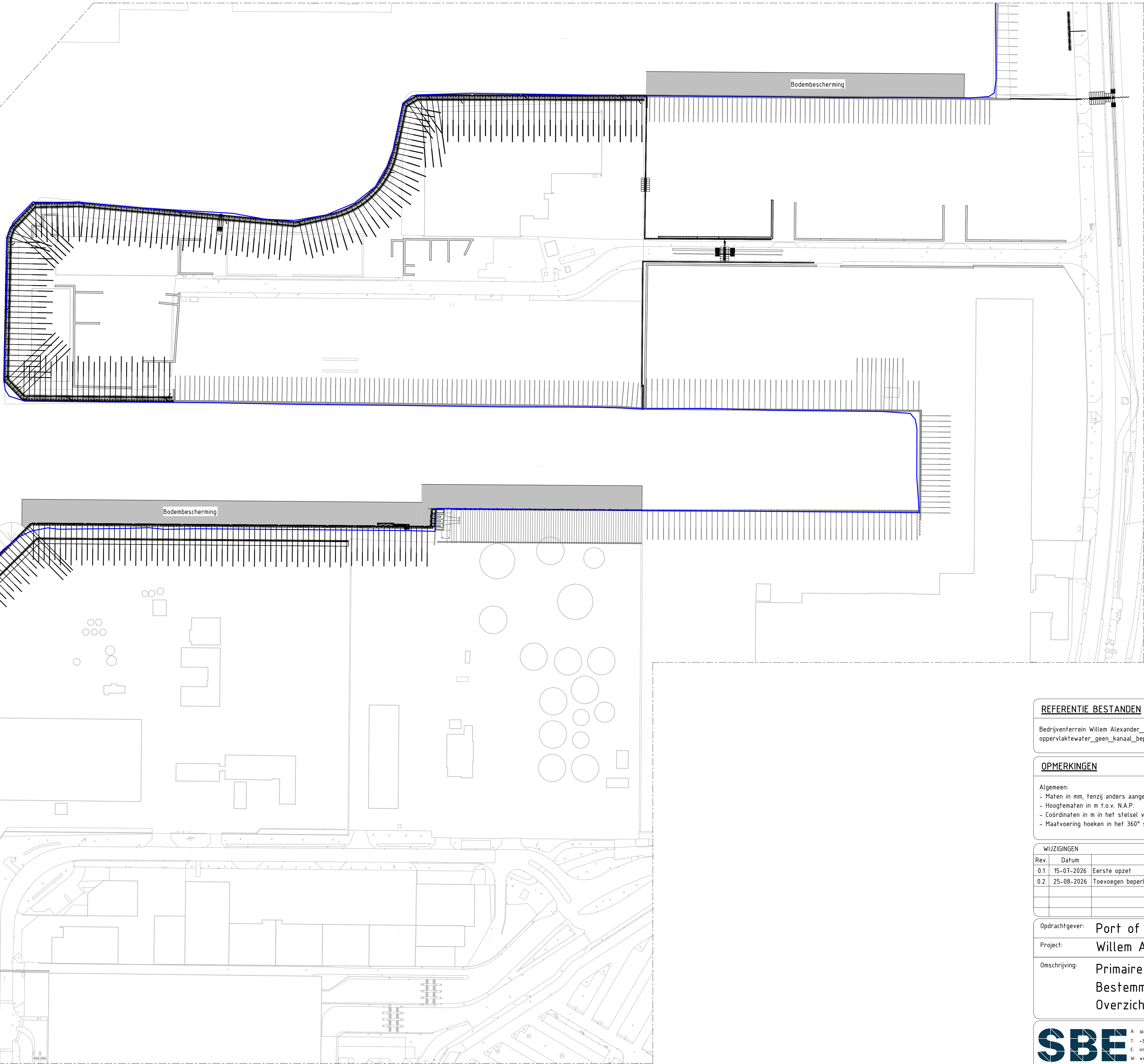
OVERZICHT PRIMAIRE WATERKERING SCHAAL: 1 : 1000
