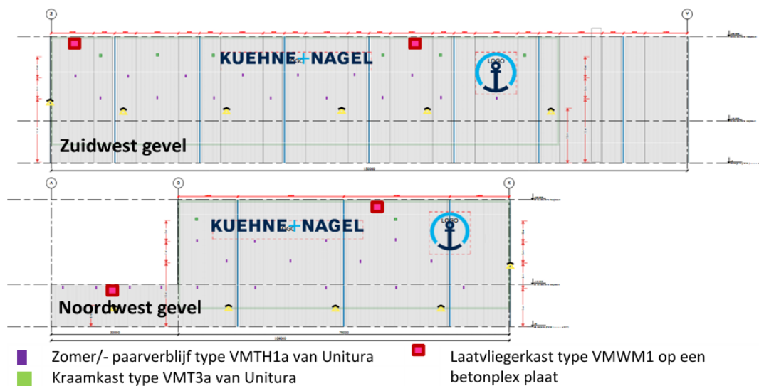
Figuur 2. Schematische weergave positionering van de tijdelijke kasten.
