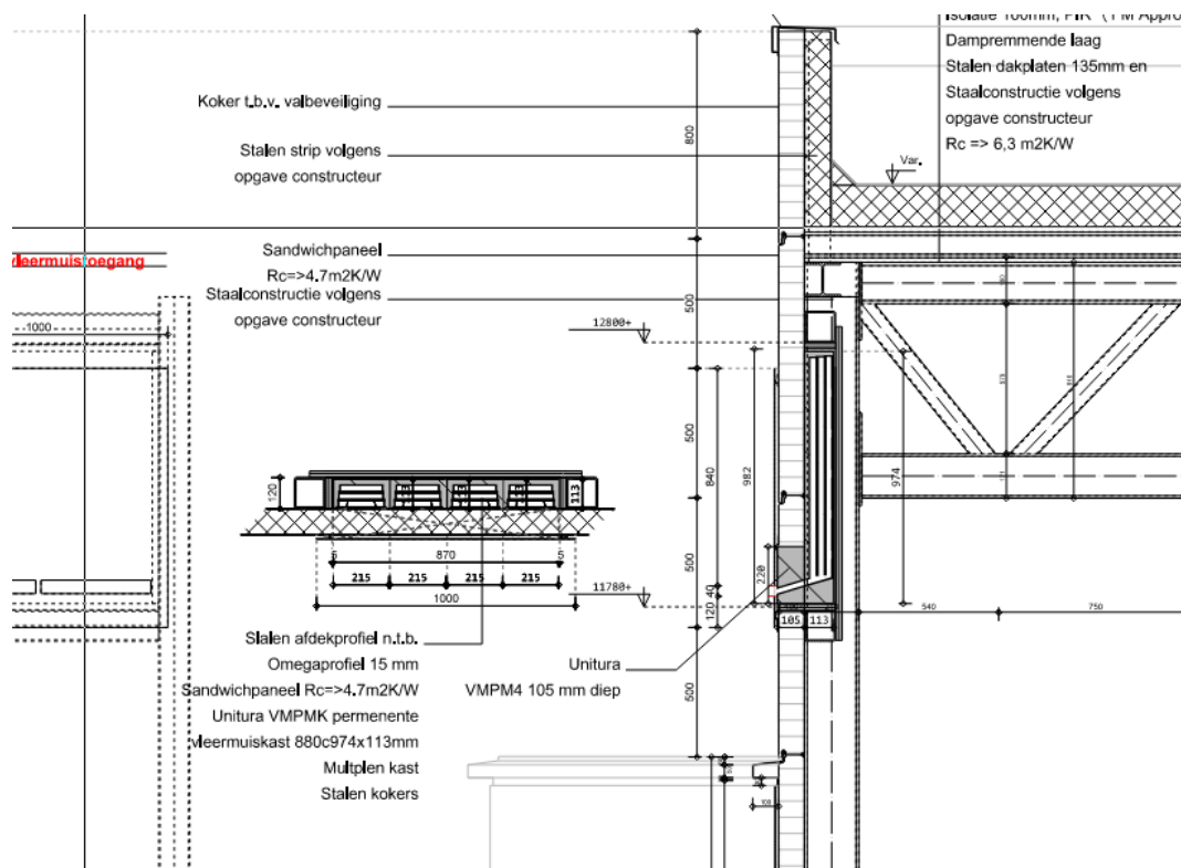
Figuur 4. Realisatie van de permanente voorzieningen.
