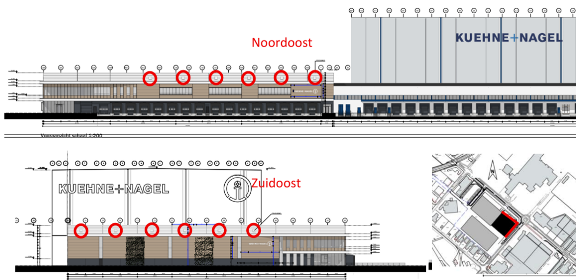
Figuur 3. Locatie van de permanente voorzieningen op de noordoost- en zuidoostgevel van het toekomstige distributiecentrum
