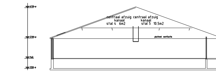
Doorsnede D-D
