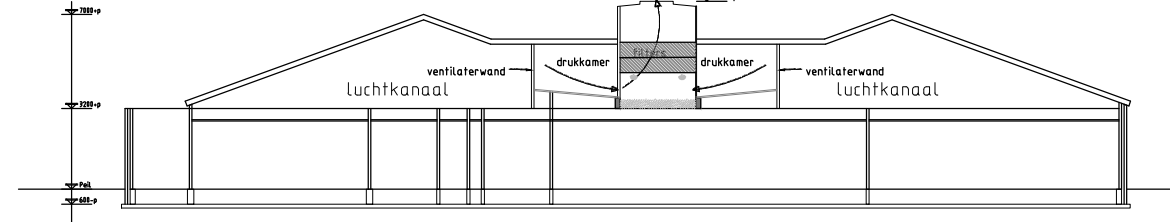
Doorsnede F-F
