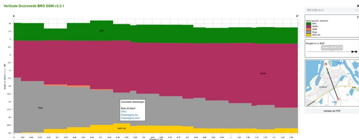
Figuur 3 Schematische weergave geologische eenheden (bron: DINOloket)
