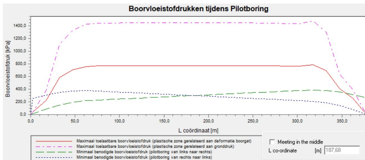
Figuur 4 Boorspoeldrukken tijdens pilotboring
