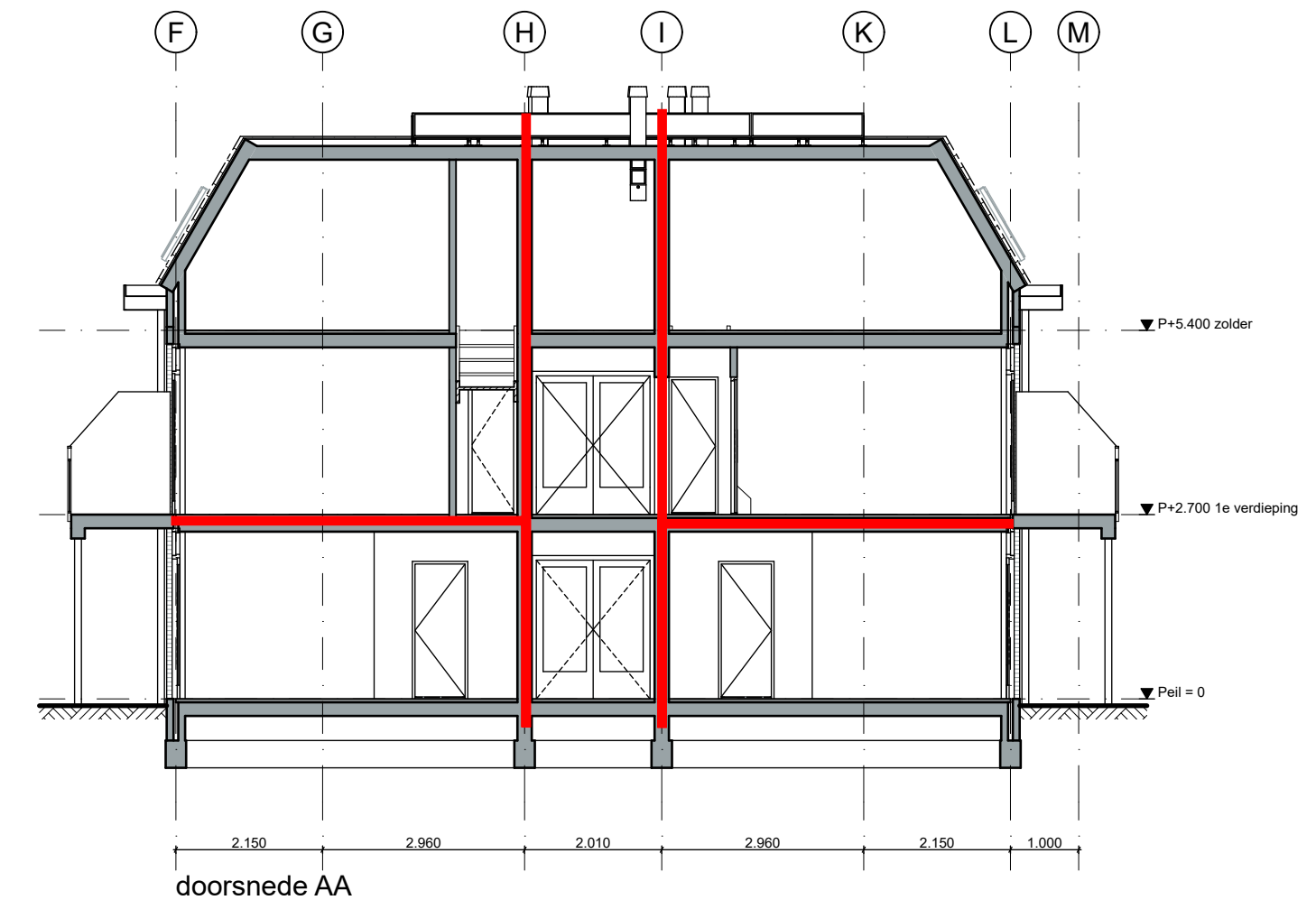
doorsnede AA
