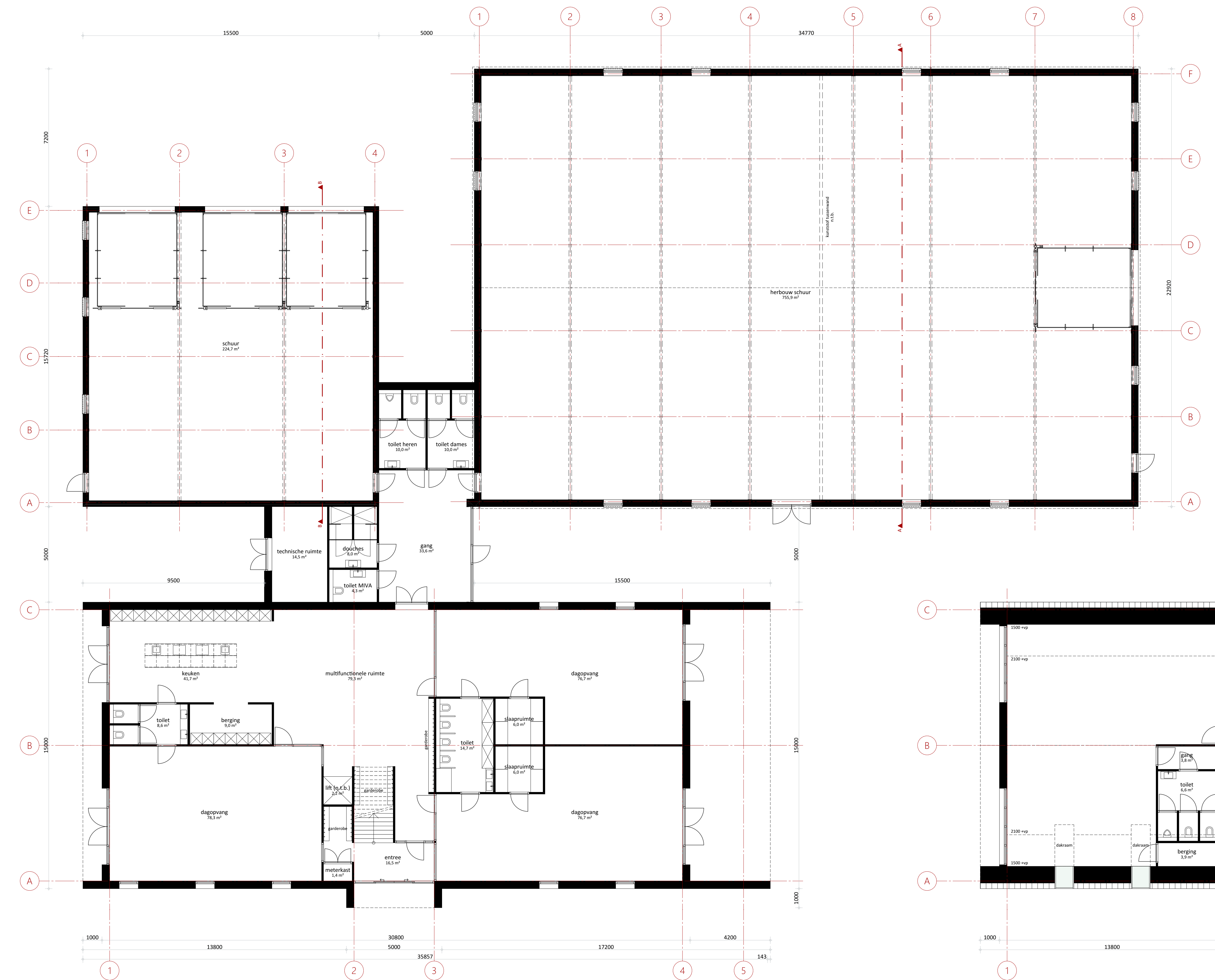
plattegrond niveau 0
