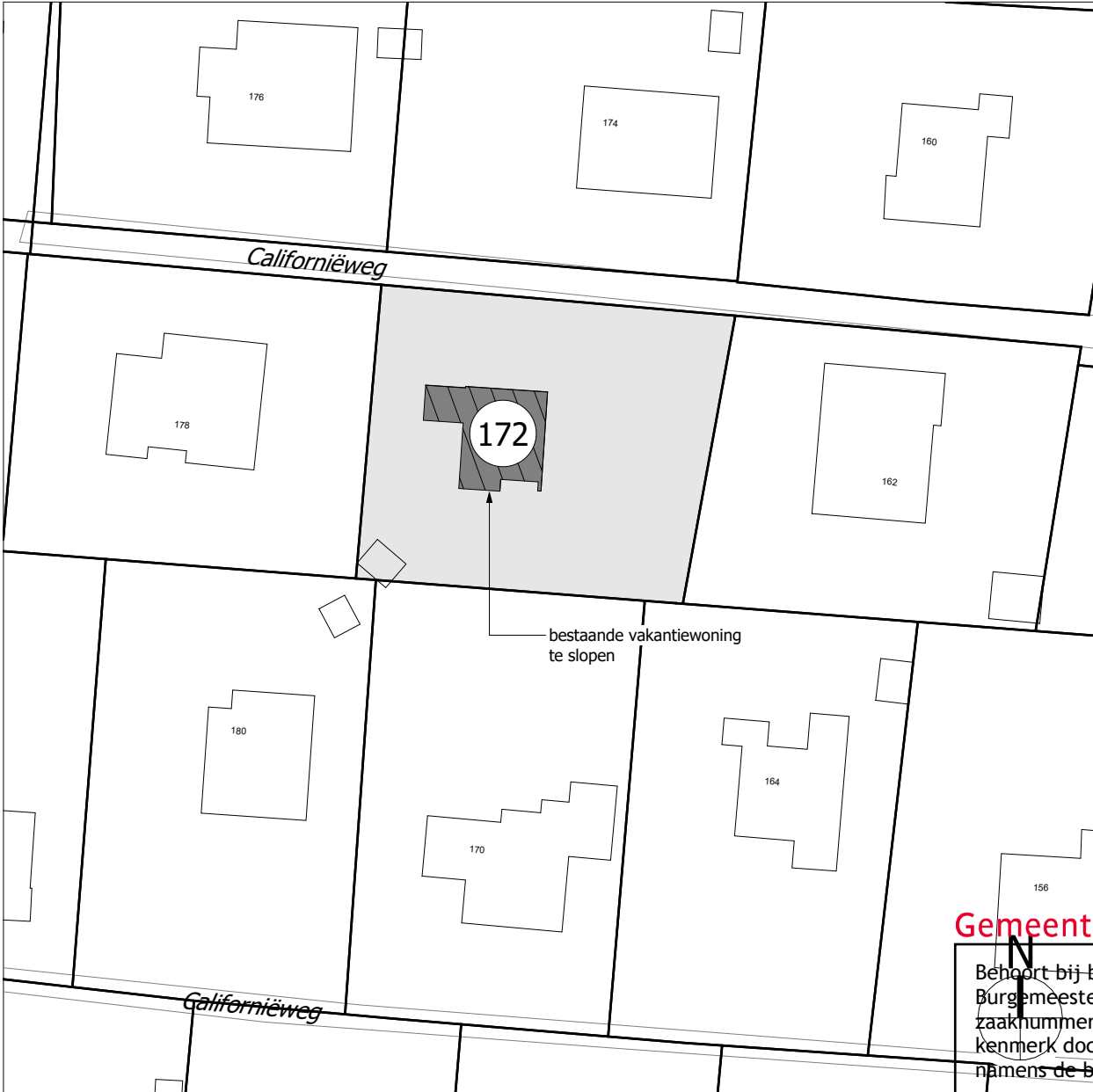
Situatie - bestaand 1 : 500
