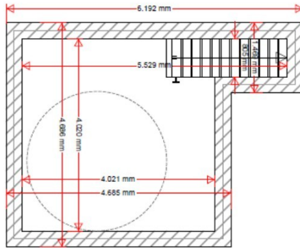
Figuur 7: Beoogde opzet vleermuiskelder
